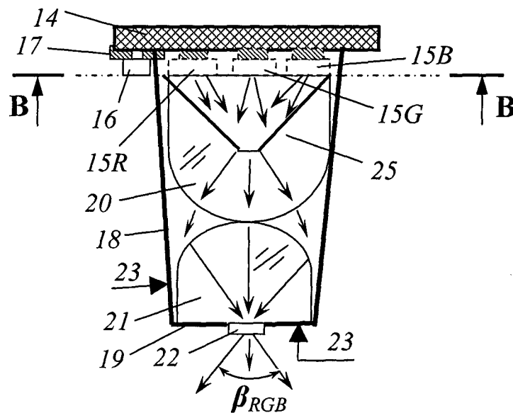
Фиг. 6 (разрез по С-С)
