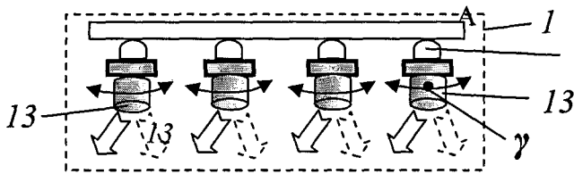
Фиг. 8 (вид В)
