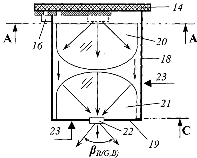
Фиг. 4 (разрез по D-D)
