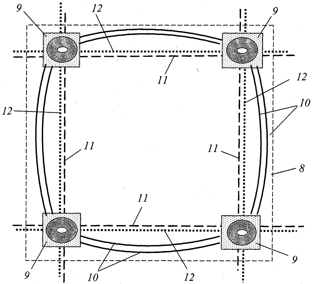
Фиг. 2 (вид А2)
