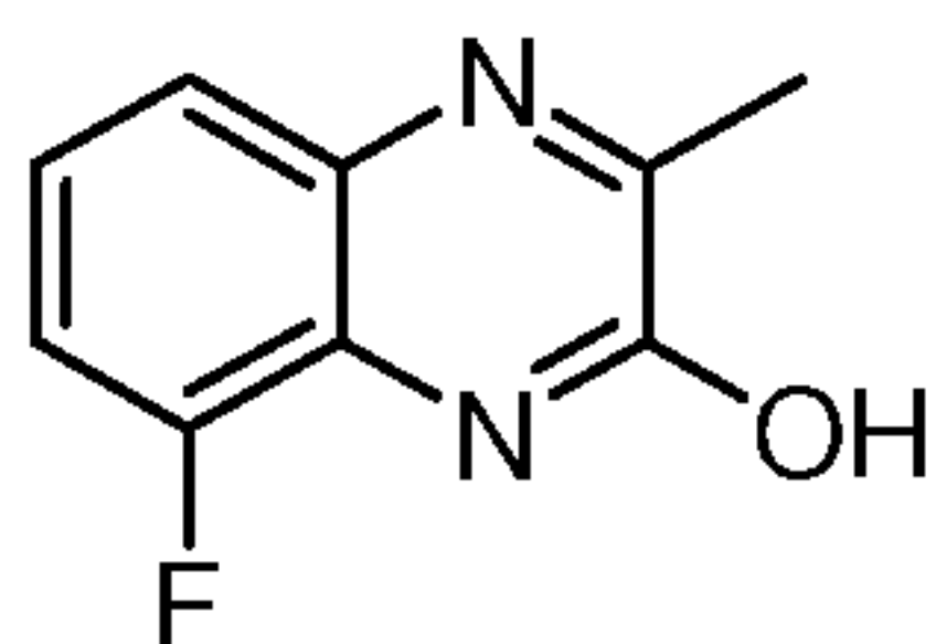
8-fluoro-3-methylquinoxalin-2-ol
