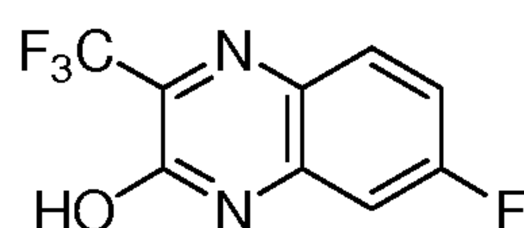
7-fluoro-3-(trifluoromethyl)quinoxalin-2-ol
