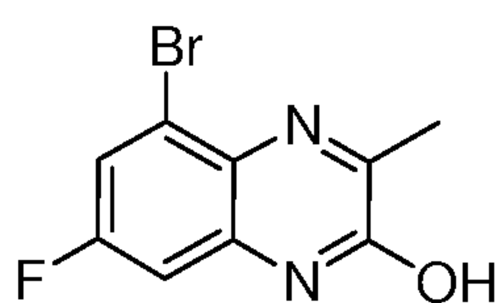
5-bromo-7-fluoro-3-methylquinoxalin-2-ol
