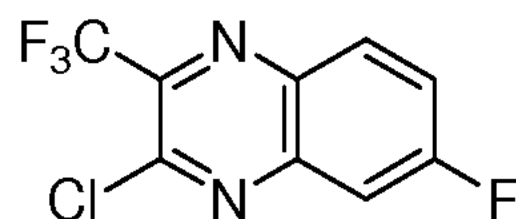
3-chloro-6-fluoro-2-(trifluoromethyl)quinoxaline
