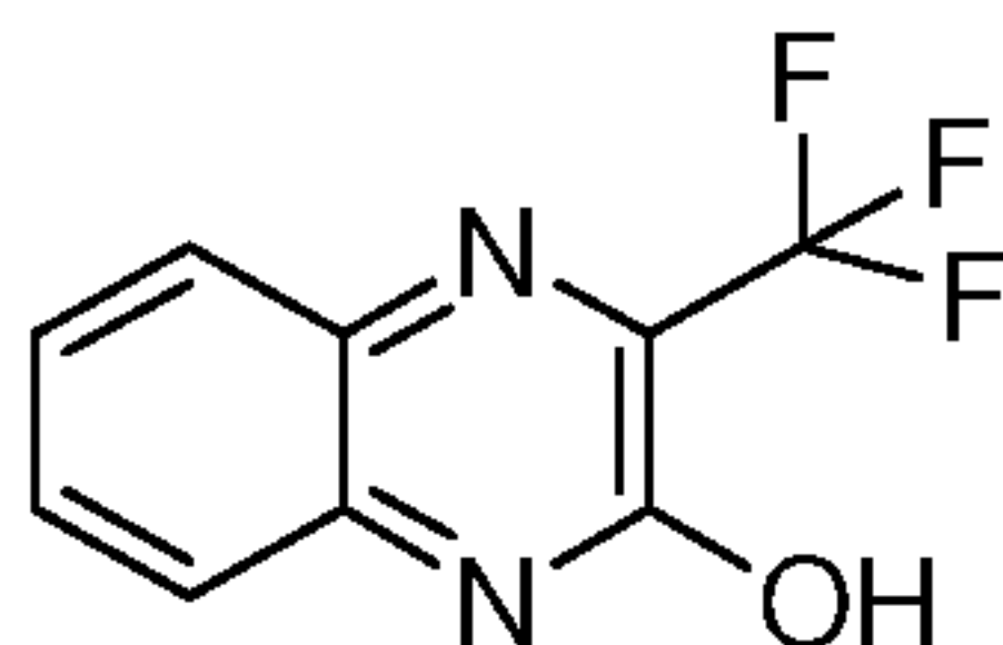
3-(trifluoromethyl)quinoxalin-2-ol
