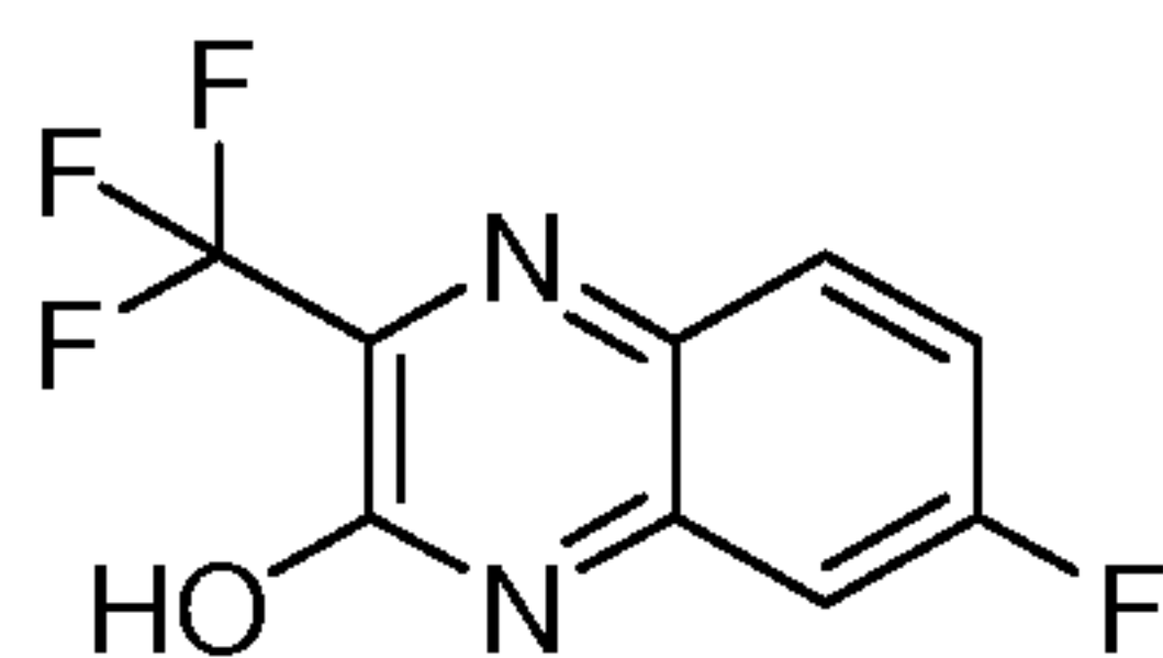
7-fluoro-3-(trifluoromethyl)quinoxalin-2-ol
