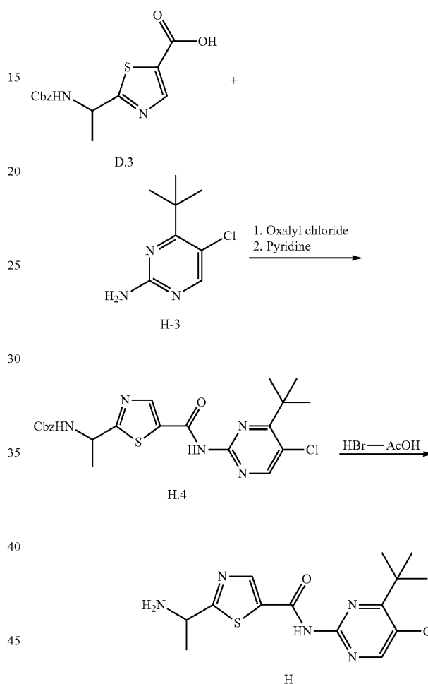
Scheme H-2.
