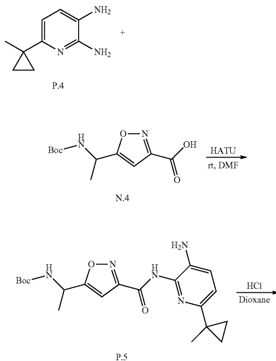
Scheme P-2.
