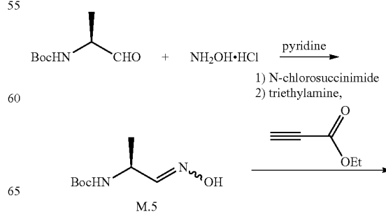
Scheme M-3.
