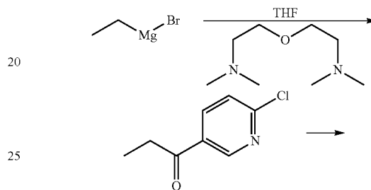
EE.1
