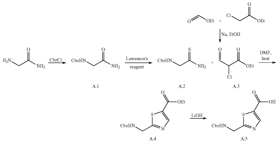
Scheme A-1.
