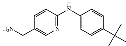
DD
