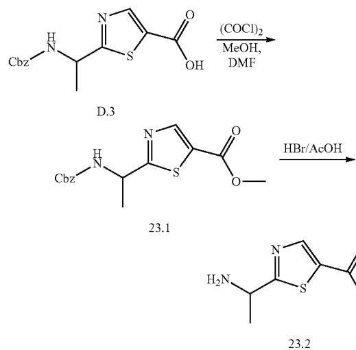
Scheme 23.
