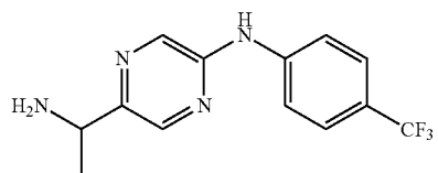
Scheme AA.
