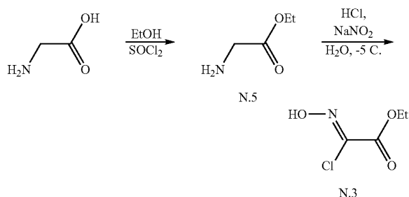
Scheme N-2.
