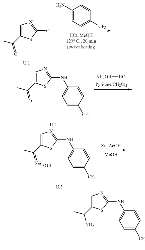
Scheme U.
