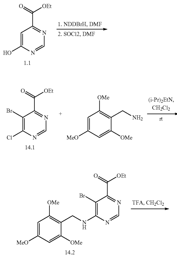
Scheme 14-1.
