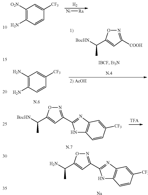
Scheme N-3.
