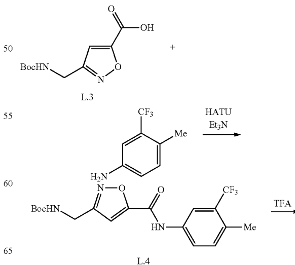
Scheme L-2.
