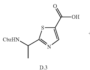
Scheme I.
