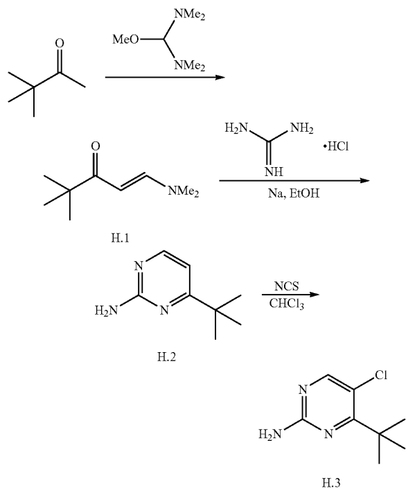
Scheme H-1.
