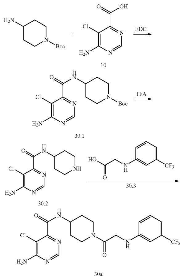
Scheme 30.
