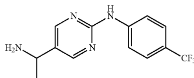
Scheme Z.
