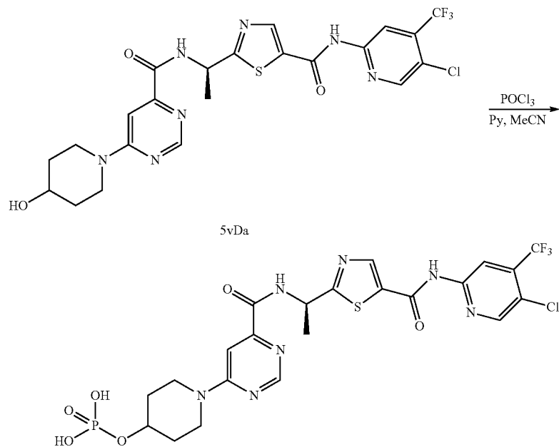
Scheme 21.
