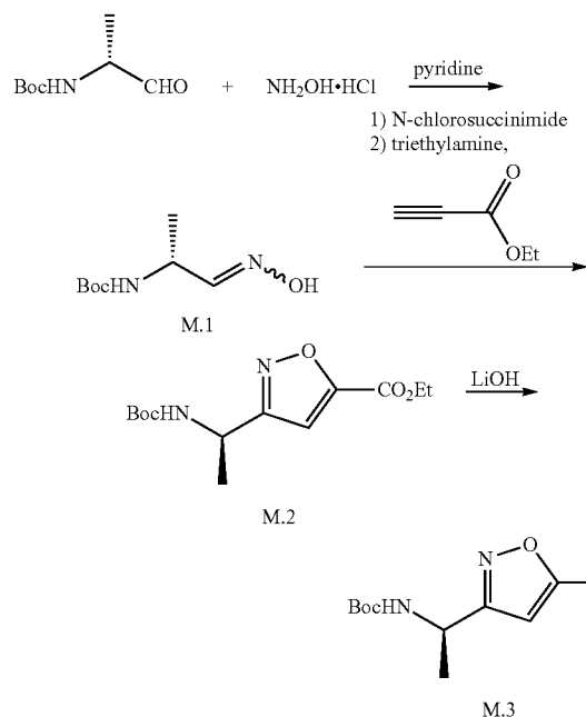
Scheme M-1.
