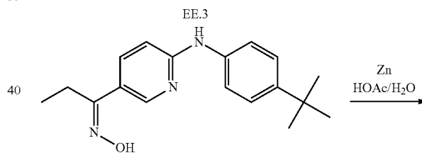
EE.4
