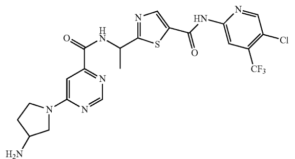
19jjD
