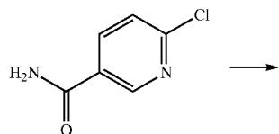
DD.1
