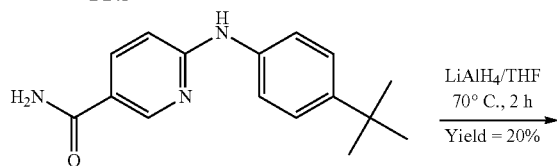
DD.2
