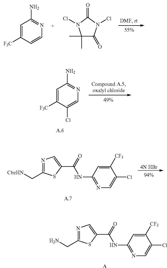
Scheme A-2.
