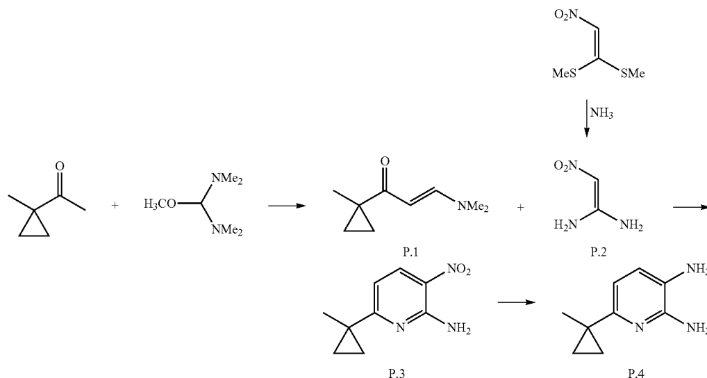
Scheme P-1.
