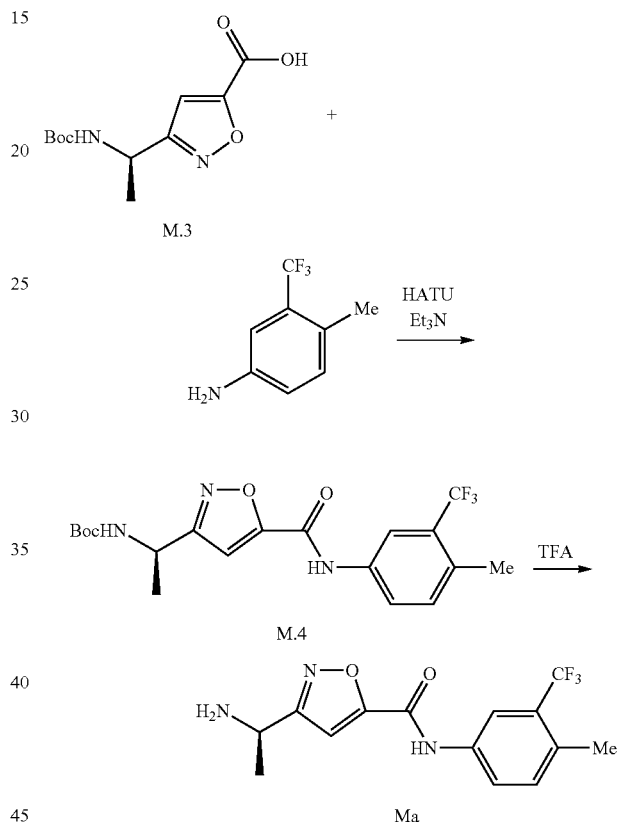
Scheme M-2.
