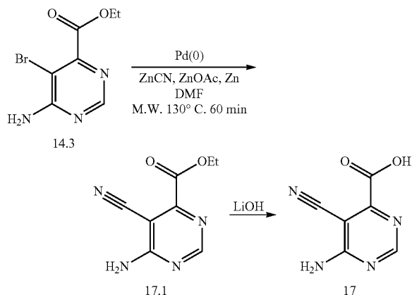
Scheme 17.
