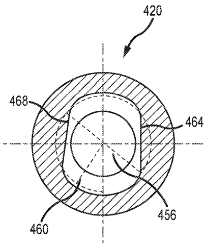
SECTION E-E FIG. 4E
