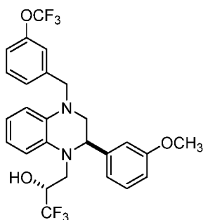
( R )- 1,1,1-trifluoro-3-(( R )-4-(3-trifluoromethoxy)benzyl)-2-(3-methoxyphenyl)-3,4-dihydroquinoxalin-1(2 H )-ylpropan-2-ol
