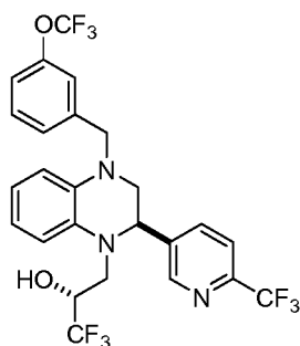
( R )-1,1,1-trifluoro-3-(( R )-4-(3-trifluoromethoxy)benzyl)-2-(6-trifluoromethyl)pyridin-3-yl)-3,4-dihydroquinoxalin-1(2 H )-yl)propan-2-ol
