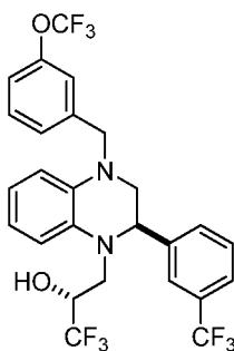
( R )-1,1,1-trifluoro-3-(( R )-4-(3-trifluoromethoxy)benzyl)-2-(3-(trifluoromethyl)phenyl)-3,4-dihydroquinoxalin-1(2 H )-ylpropan-2-ol
