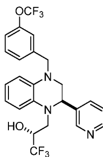
( R )- 1,1,1-trifluoro-3-(( R )-2-(pyridine-3-yl)-4-(3-trifluoromethoxy)benzyl)-3,4-dihydroquinoxalin-1(2 H )-ylpropan-2-ol
