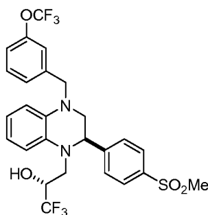
( R )- 1,1,1-trifluoro-3-(( R )-2-(4-methylsulfonyl)phenyl)-4-(3-trifluoromethoxy)benzyl)-3,4-dihydroquinoxalin-1(2 H )-ylpropan-2-ol
