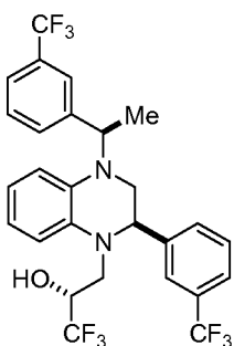
( R )-1,1,1-trifluoro-3-(( R )-2-(3-(trifluoromethyl)phenyl)-4-(( R )-1-(3-(trifluoromethyl)phenyl)ethyl)-3,4-dihydroquinoxalin-1(2 H )-yl)propan-2-ol
