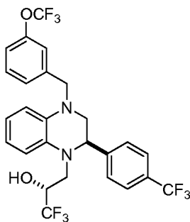
( R )-1,1,1-trifluoro-3-(( R )-4-(3-trifluoromethoxy)benzyl)-2-(4-(trifluoromethyl)phenyl)-3,4-dihydroquinoxalin-1(2 H )-ylpropan-2-ol
