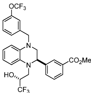
Methyl-3-(( R )-1-( R -3,3,3-trifluoro-2-hydroxypropyl)-4-(3-trifluoromethoxy)benzyl)-1,2,3,4-tetrahydroquinoxalin-2-yl)benzoate
