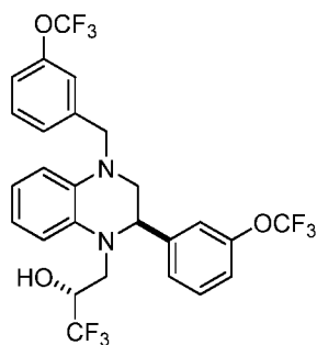
( R )- 1,1,1-trifluoro-3-(( R )-4-(3-trifluoromethoxy)benzyl)-2-(3-trifluoromethoxyphenyl)-3,4-dihydroquinoxalin-1(2 H )-ylpropan-2-ol
