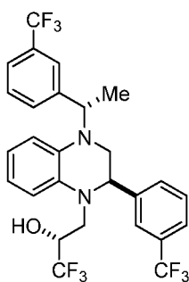
( R )-1,1,1-trifluoro-3-(( R )-2-(3-(trifluoromethyl)phenyl)-4-(( S )-1-(3-(trifluoromethyl)phenyl)ethyl)-3,4-dihydroquinoxalin-1(2 H )-yl)propan-2-ol
