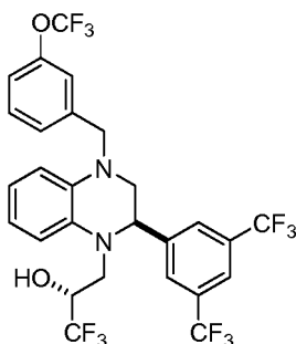
( R )- 1,1,1-trifluoro-3-(( R )-2-(3,5-bis-trifluoromethylphenyl)4-(3-trifluoromethoxy)benzyl)-3,4-dihydroquinoxalin-1(2 H )-ylpropan-2-ol
