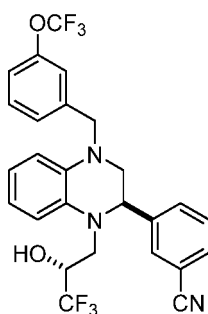
( R )- 1,1,1-trifluoro-3-(( R )-2-(3-cyanophenyl)4-(3-trifluoromethoxy)benzyl)-3,4-dihydroquinoxalin-1(2 H )-ylpropan-2-ol
