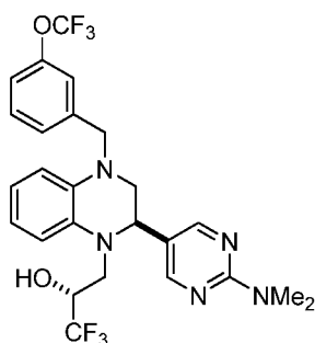
( R )-3-(( R )-2(2-dimethylamino)pyrimidin-5-yl)-4-(3-trifluoromethoxy)benzyl)-3,4-dihydroquinoxalin-1(2 H )-yl)-1,1,1-trifluoropropan-2-ol
