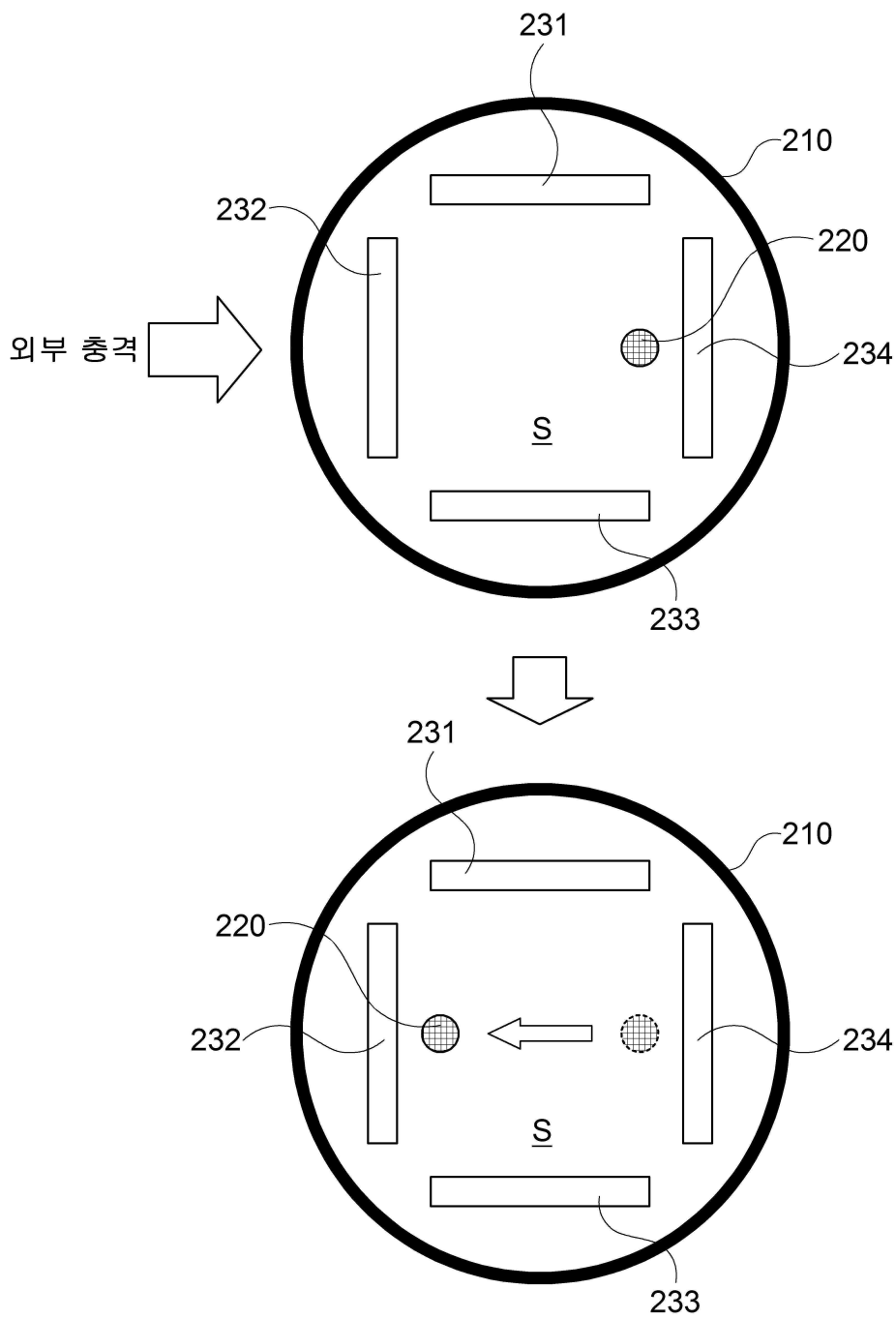
도면4
