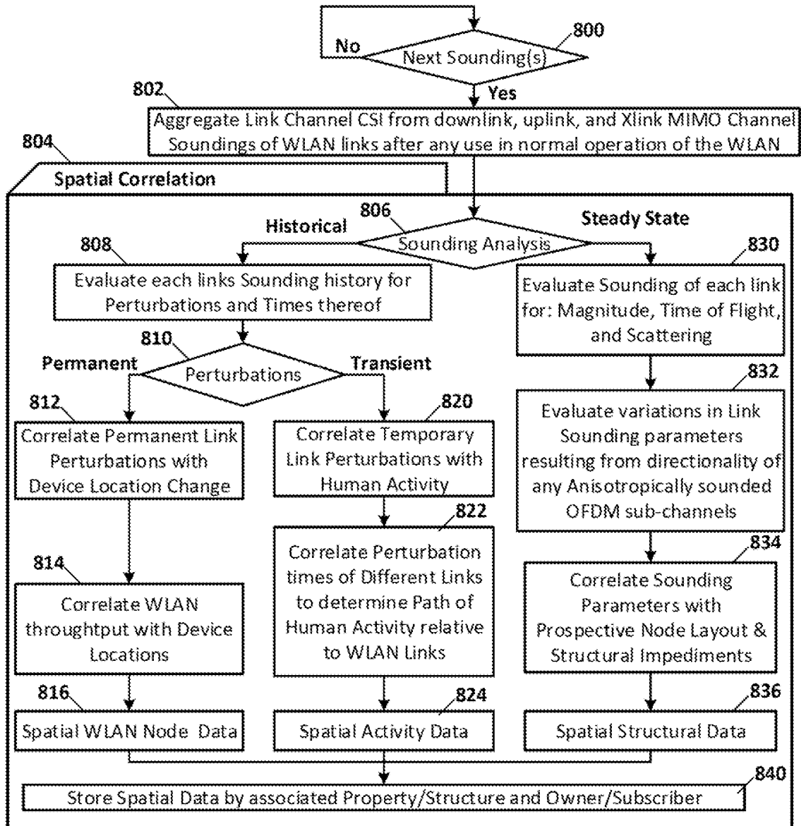
FIG. 8A WLAN Spatial Diagnostics
