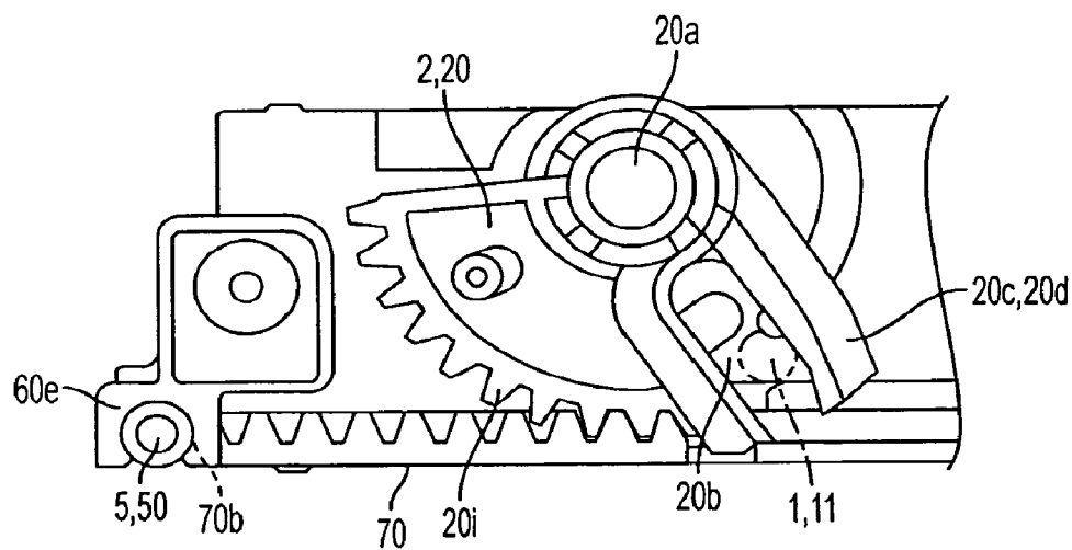
FIG. 7B
