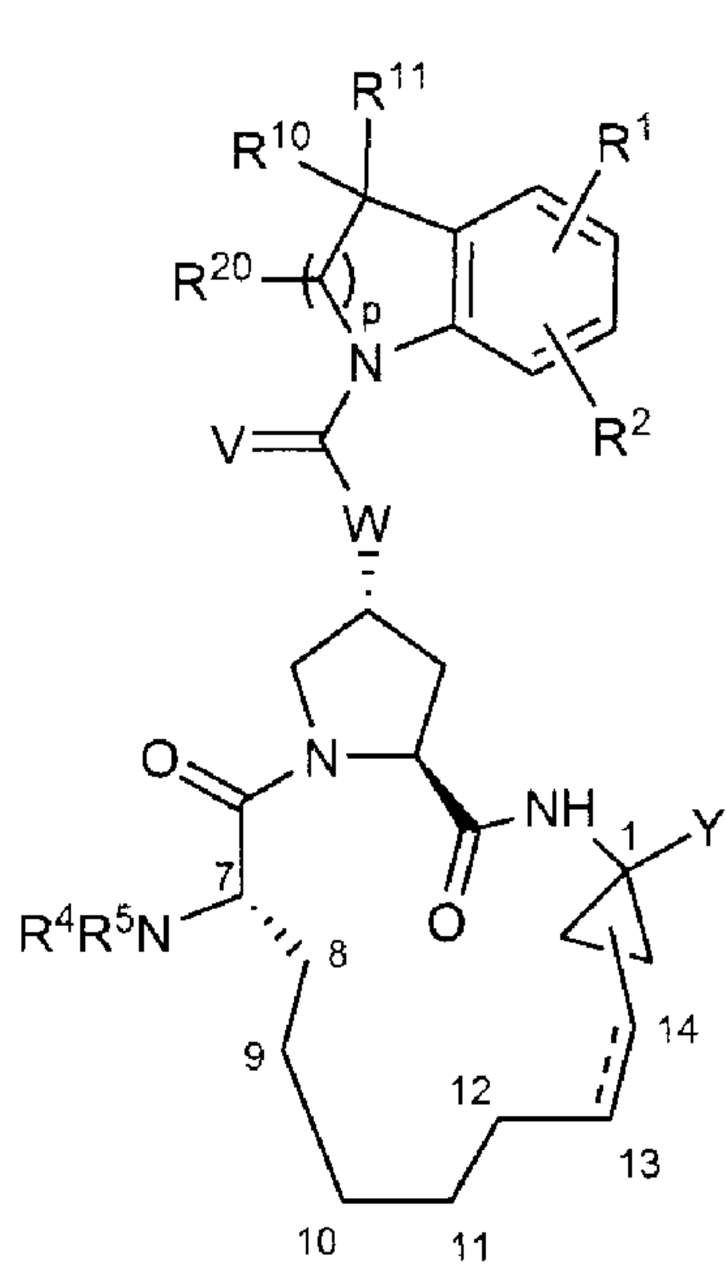
VIII
