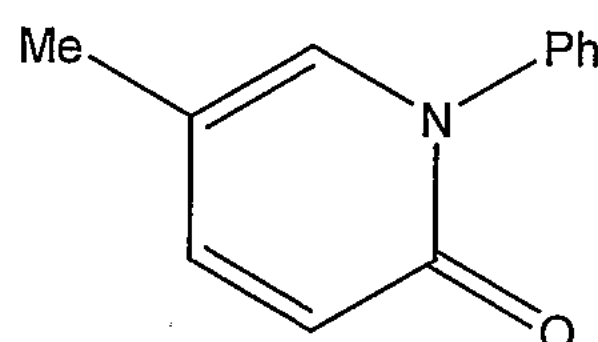
Pirfenidone analogs
