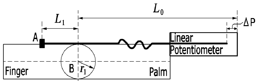
(d) Necessity of a spring
