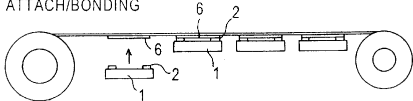
DIE ATTACH/BONDING
