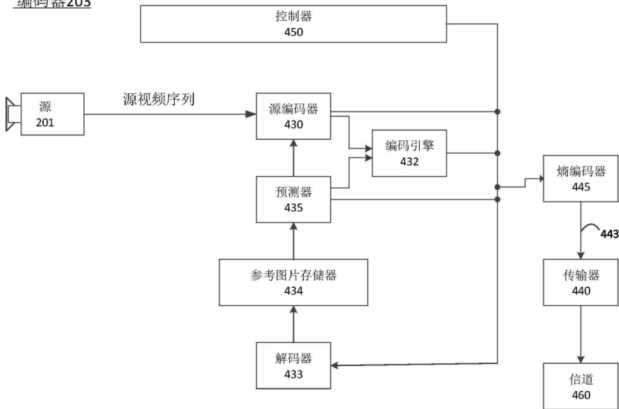
编码器203
