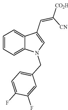
(E)-2-Cyano-3-(1-(3,4-difluorobenzyl)-1H-indol-3-yl)acrylic Acid (JXL016)
