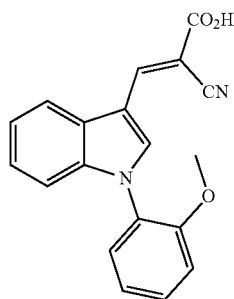
(E)-2-Cyano-3-(1-(2-methoxyphenyl)-1H-indol-3-yl) acrylic Acid (JXL014)
