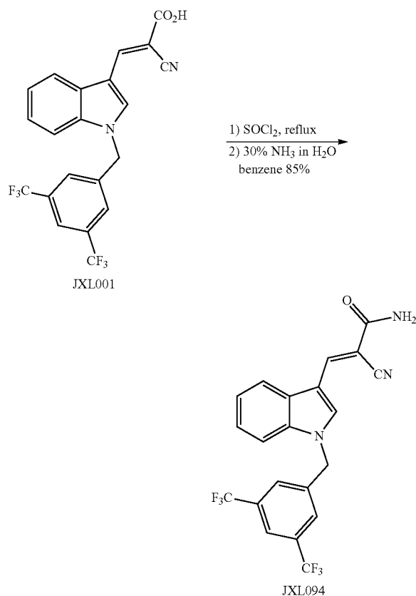
(E)-3-(1-(3,5-Bis(trifluoromethyl)benzyl)-1H-indol-3-yl)-2-cyanoacrylamide (JXL094)
