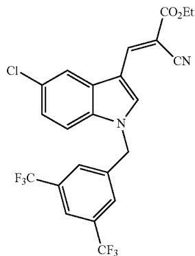
Ethyl (E)-3-(1-(3,5-bis(trifluoromethyl)benzyl)-5-chloro-1H-indol-3-yl)-2-cyanoacrylate (JXL089)
