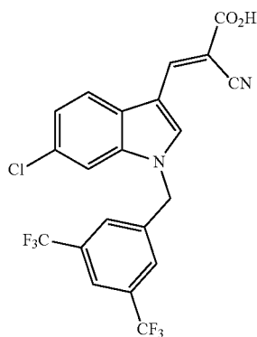
(E)-3-(1-(3,5-Bis(trifluoromethyl)benzyl)-6-chloro-1H-indol-3-yl)-2-cyanoacrylic Acid (JXL063)
