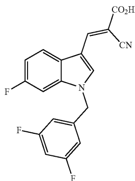
(E)-2-Cyano-3-(1-(3,5-difluorobenzyl)-6-fluoro-1H-indol-3-yl)acrylic Acid (JXL040)
