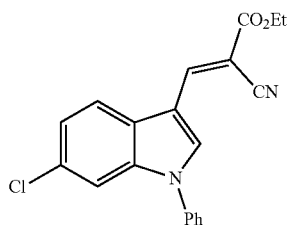
Ethyl (E)-3-(6-chloro-1-phenyl-1H-indol-3-yl)-2-cyanoacrylate (JXL005)
