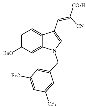
(E)-3-(6-(Benzyloxy)-1-(3,5-bis(trifluoromethyl)benzyl)-1H-indol-3-yl)-2-cyanoacrylic Acid (JXL058)
