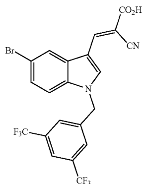
(E)-3-(1-(3,5-Bis(trifluoromethyl)benzyl)-5-bromo-1H-indol-3-yl)-2-cyanoacrylic Acid (JXL061)
