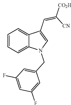
(E)-2-Cyano-3-(1-(3,5-difluorobenzyl)-1H-indol-3-yl)acrylic Acid (JXL017)
