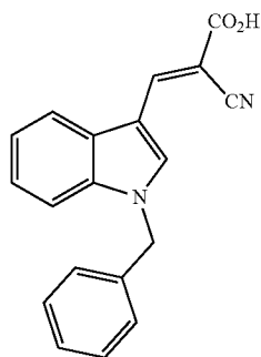
(E)-3-(1-Benzyl-1H-indol-3-yl)-2-cyanoacrylic Acid (JXL019)
