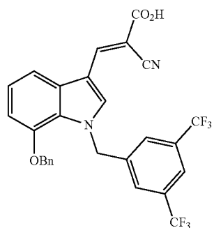
(E)-3-(7-(Benzyloxy)-1-(3,5-bis(trifluoromethyl)benzyl)-1H-indol-3-yl)-2-cyanoacrylic Acid (JXL059)
