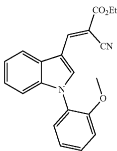
Ethyl (E)-2-cyano-3-(1-(2-methoxyphenyl)-1H-indol-3-yl)acrylate (JXL006)
