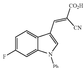
(E)-2-Cyano-3-(6-fluoro-1-phenyl-1H-indol-3-yl) acrylic Acid (JXL027)
