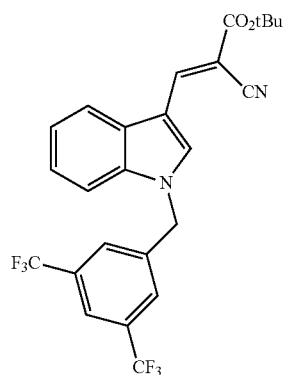
tert-Butyl (E)-3-(1-(3,5-bis(trifluoromethyl)benzyl)-1H-indol-3-yl)-2-cyanoacrylate (JXL068)
