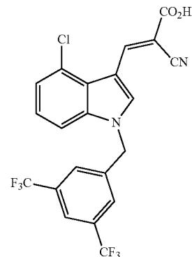
(E)-3-(1-(3,5-Bis(trifluoromethyl)benzyl)-4-chloro-1H-indol-3-yl)-2-cyanoacrylic Acid (JXL050)
