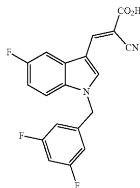
(E)-2-Cyano-3-(1-(3,5-difluorobenzyl)-5-fluoro-1H-indol-3-yl)acrylic Acid (JXL037)
