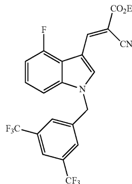
Ethyl (E)-3-(1-(3,5-bis(trifluoromethyl)benzyl)-4-fluoro-1H-indol-3-yl)-2-cyanoacrylate (JXL066)
