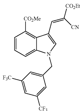
Methyl (E)-1-(3,5-bis(trifluoromethyl)benzyl)-3-(2-cyano-3-ethoxy-3-oxoprop-1-en-1-yl)-1H-indole-4-carboxylate (JXL091)
