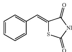
(Z)-5-Benzylidenethiazolidine-2,4-dione (JXL074)
