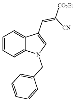
Ethyl (E)-3-(1-benzyl-1H-indol-3-yl)-2-cyanoacrylate (JXL018)
