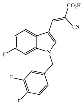
(E)-2-Cyano-3-(1-(3,4-difluorobenzyl)-6-fluoro-1H-indol-3-yl)acrylic Acid (JXL039)
