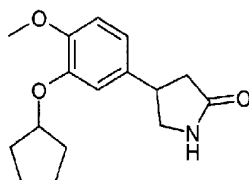
rolipram
