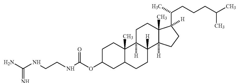
CHOL-GUA
