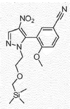
4-methoxy-3-(4-nitro-1-(2-((trimethylsilyl)methoxy)ethyl)-1H-pyrazol-5-yl)benzonitrile
