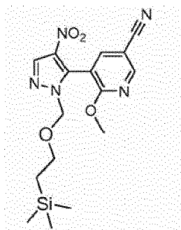
6-Methoxy-5-(4-nitro-1-((2-(trimethylsilyl)ethoxy)methyl)-1H-pyrazol-5-yl)nicotinonitrile
