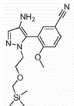
3-(4-amino-1-(2-((trimethylsilyl)methoxy)ethyl)-1H-pyrazol-5-yl)-4-methoxybenzonitrile
