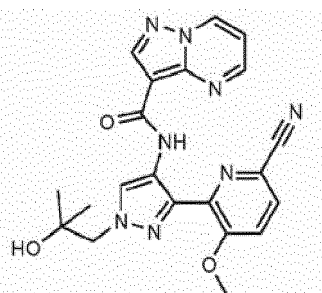
N-(3-(6-cyano-3-methoxypyridin-2-yl)-1-(2-hydroxy-2-methylpropyl)-1H-pyrazol-4-yl)pyrazolo[1,5-a]pyrimidine-3-carboxamide
