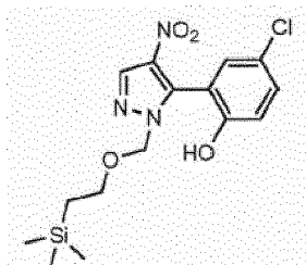
4-chloro-2-(4-nitro-1-((2-(trimethylsilyl)ethoxy)methyl)-1H-pyrazol-5-yl)phenol
