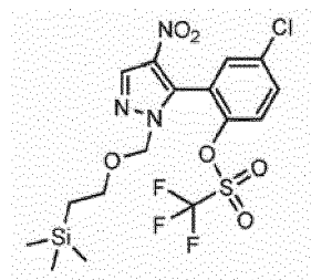
4-chloro-2-(4-nitro-1-((2-(trimethylsilyl)ethoxy)methyl)-1H-pyrazol-5-yl)phenyl trifluoromethanesulfonate
