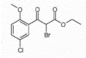
ethyl 2-bromo-3-(5-chloro-2-methoxyphenyl)-3-oxopropanoate
