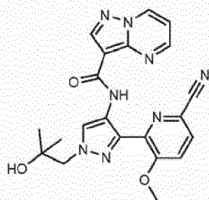
N-(3-(6-cyano-3-methoxypyridin-2-yl)-1-(2-hydroxy-2-methylpropyl)-1H-pyrazol-4-yl)pyrazolo[1,5-a]pyrimidine-3-carboxamide
