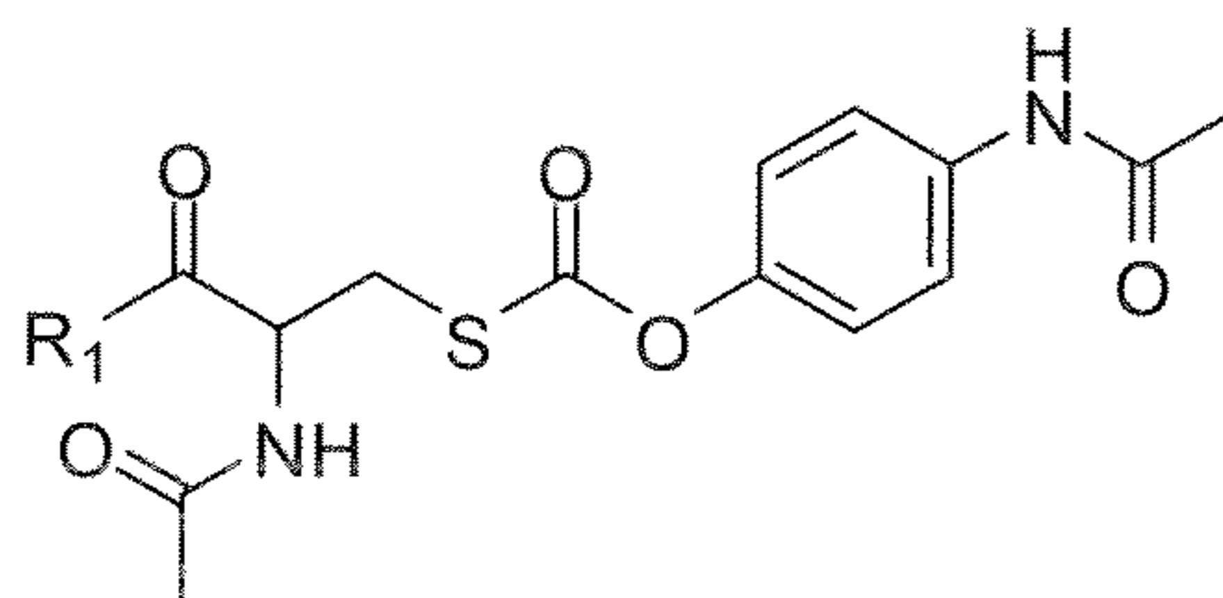
(XVII)
