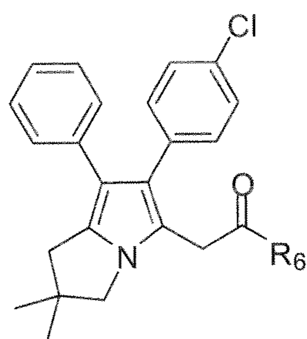
(VII)
