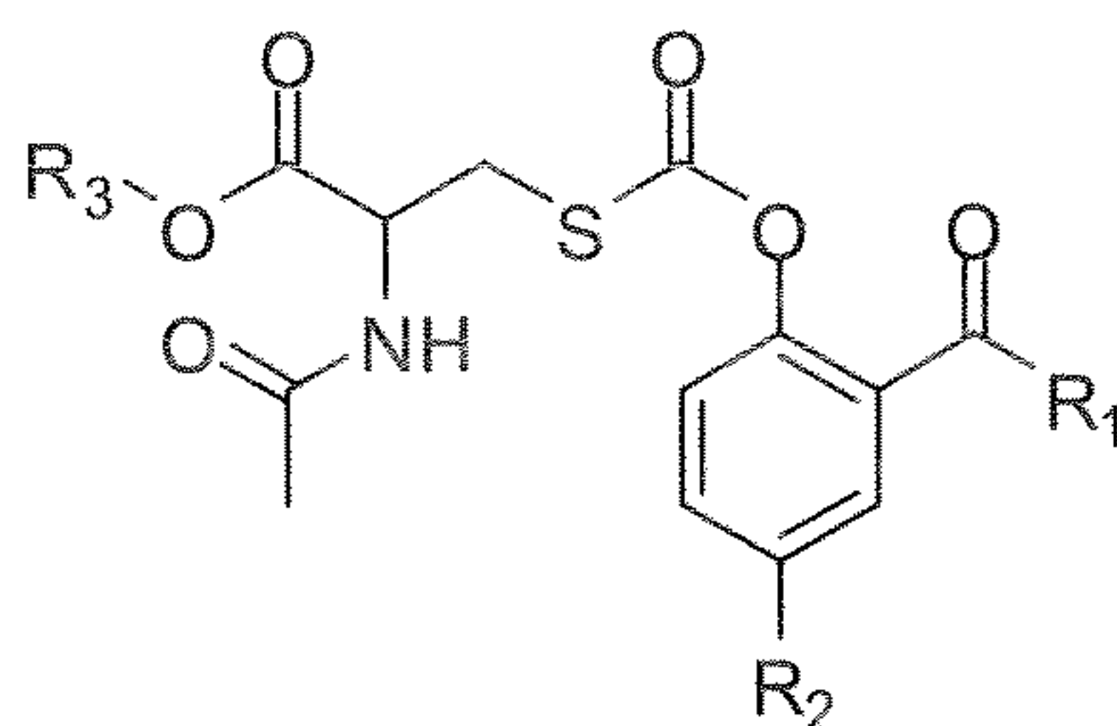
(XIV)
