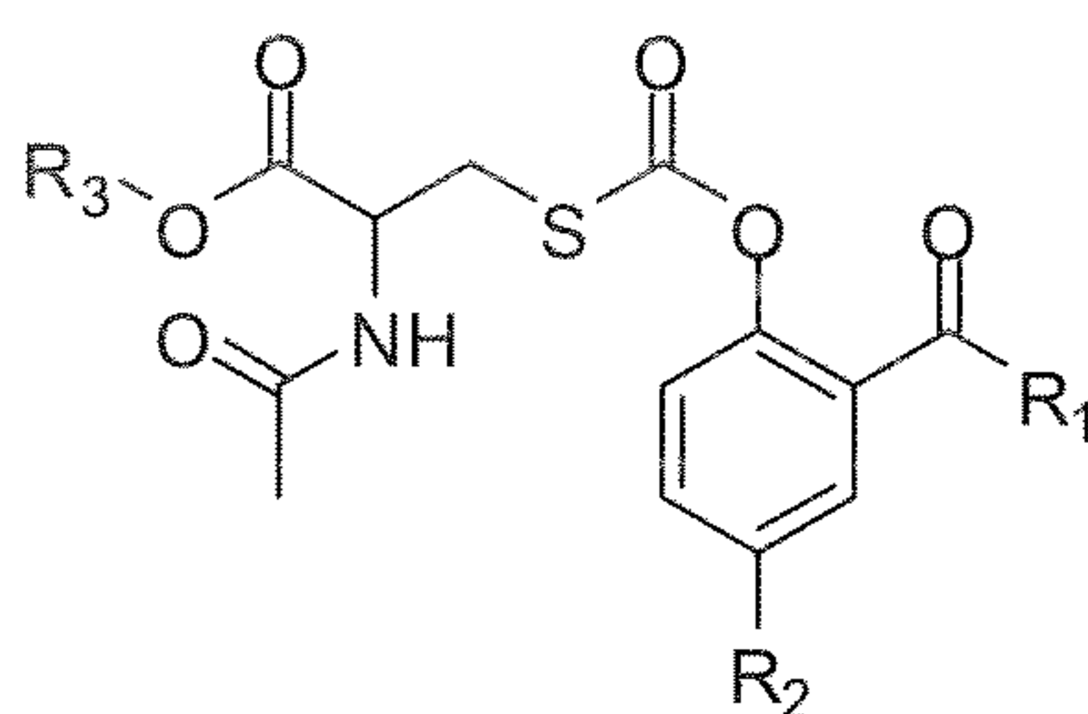
(XIV)
