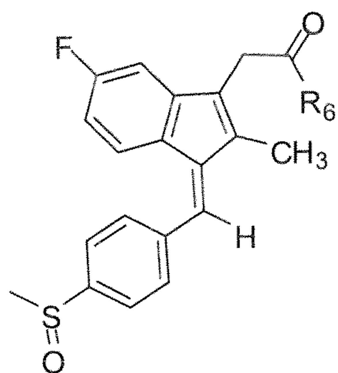
(VIII)
