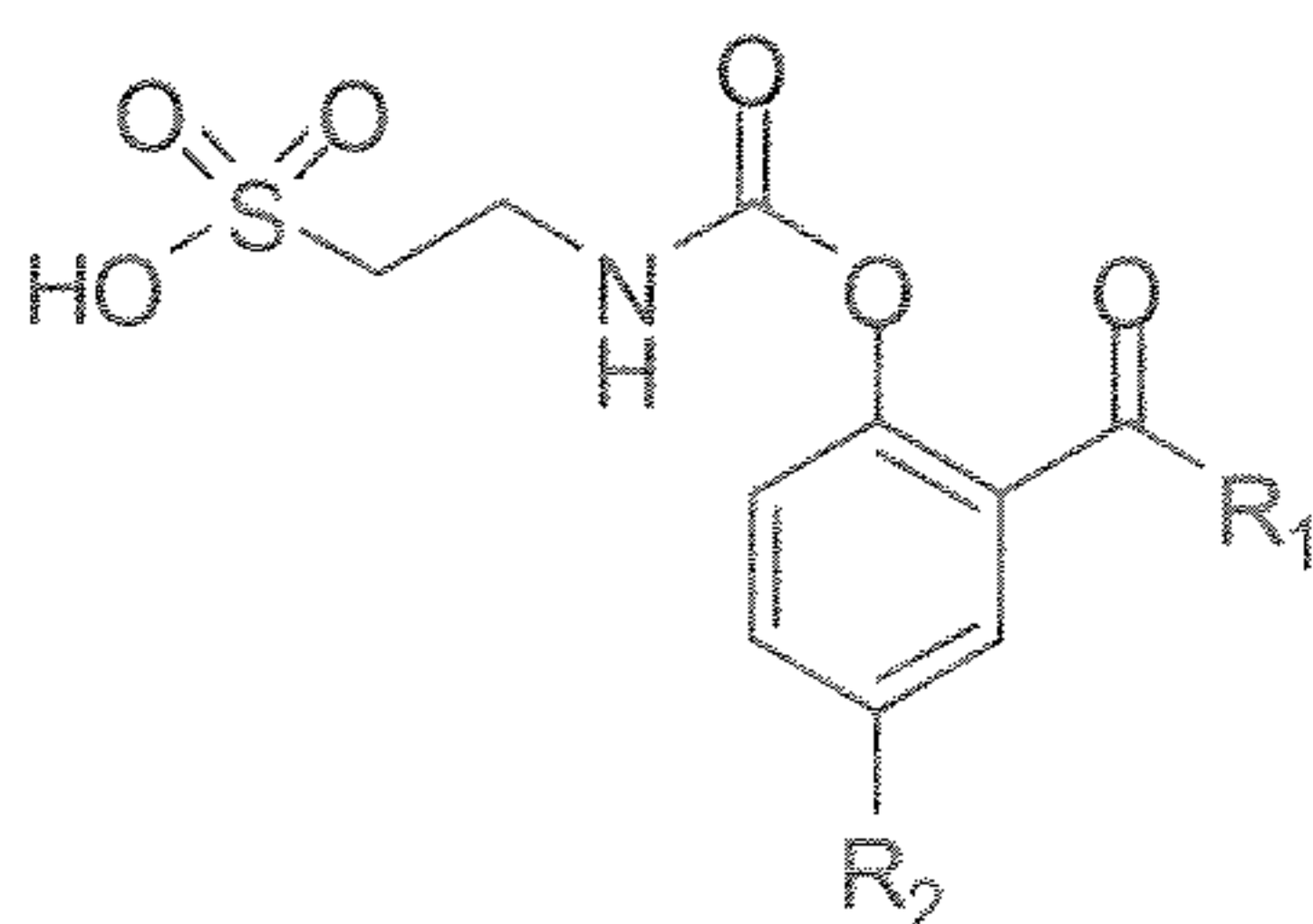
(XV)
