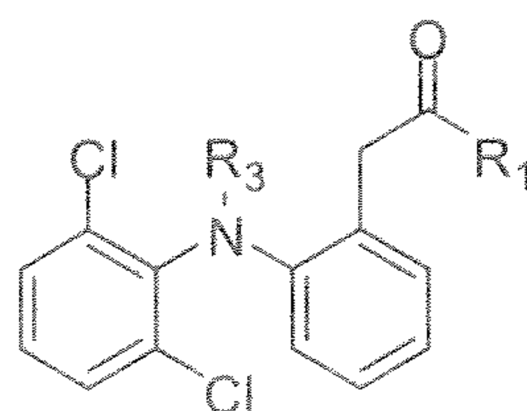
(XVIII)
