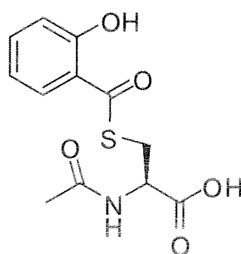
Salnacedin
