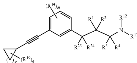
Formula (D)
