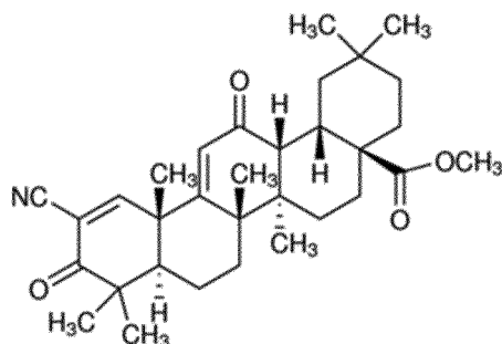
CDDO-Me
