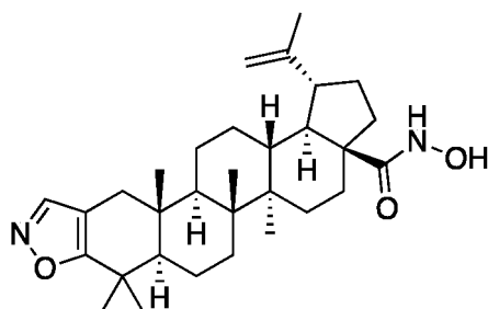
Lup-2-eno[2,3-d]isoxazol-N-hydroxy-28-amide
