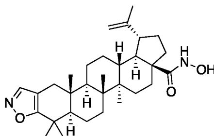
Lup-2-éno[2,3-d]isoxazol-N-hydroxy-28-amide
