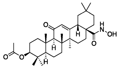
(3β) 3-acétyloxy-11-oxo-oléan-12-ène-N-hydroxy-28-amide ;
