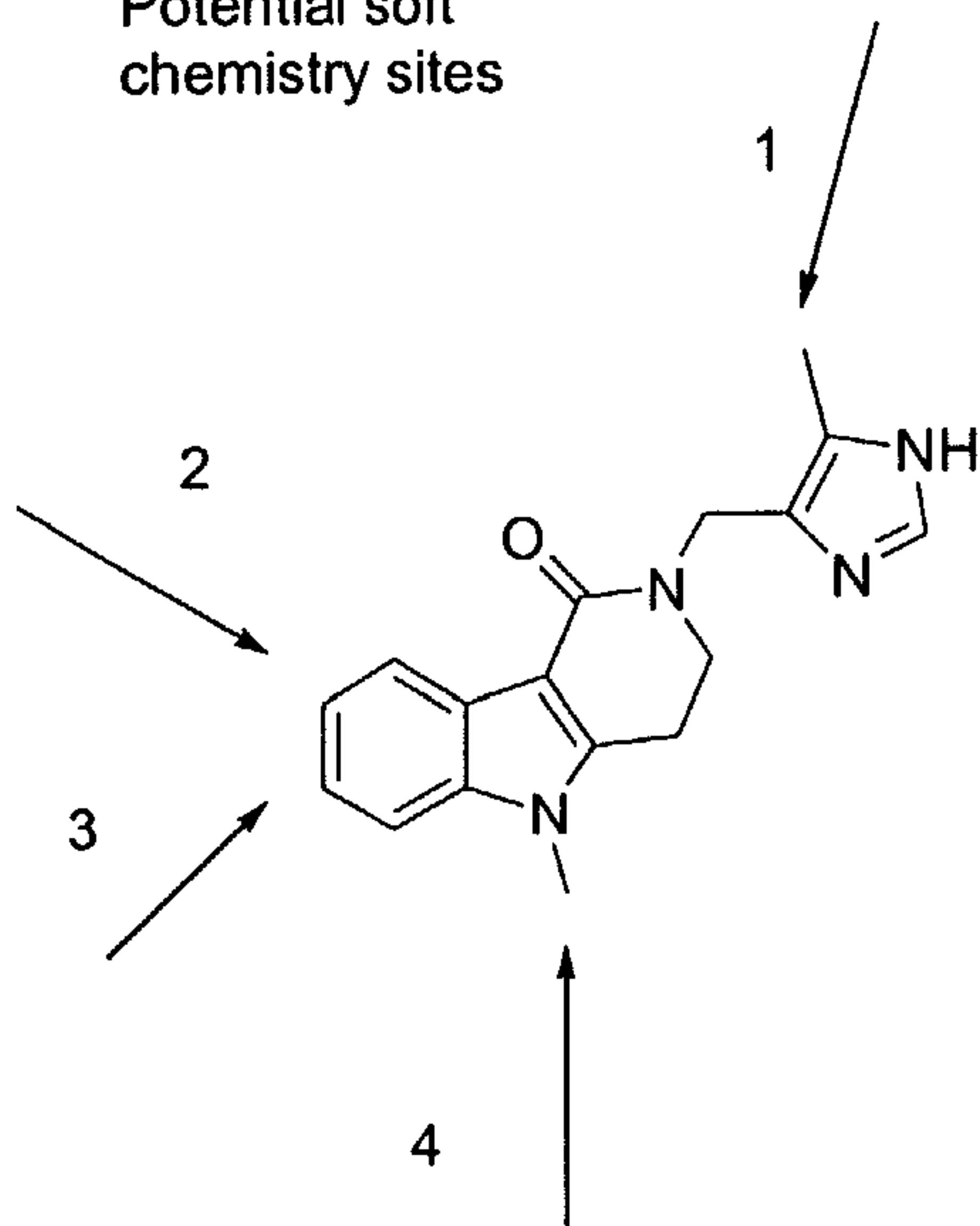
Alosetron
