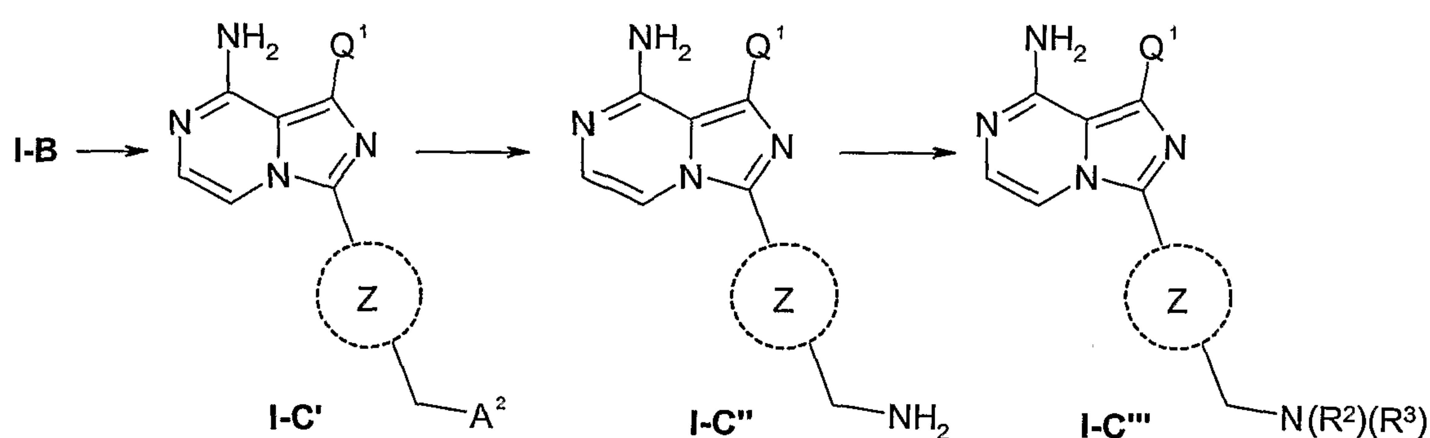
Scheme 8a
