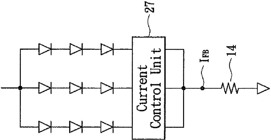
FIG. 12C
