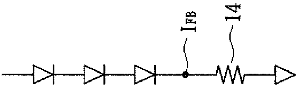
FIG. 12A
