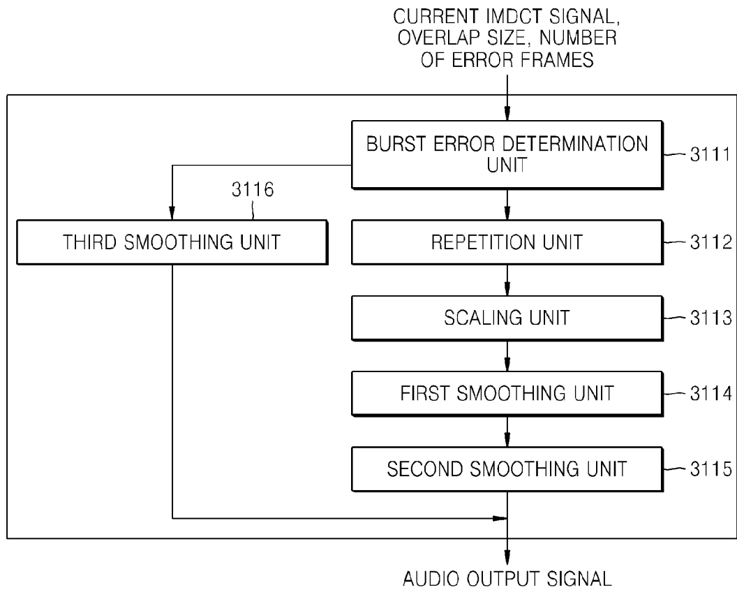
FIG. 31A
