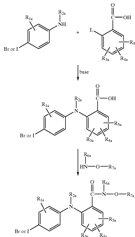
Scheme 1a
