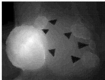
pxint1, Cy-5ex, Cy5em
