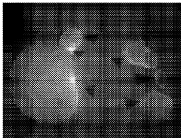
pxint1, Cy-5ex, Cy7em
