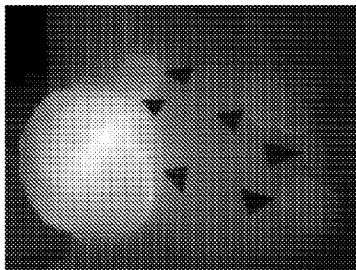
pxint1, Cy-5ex, Cy5em
