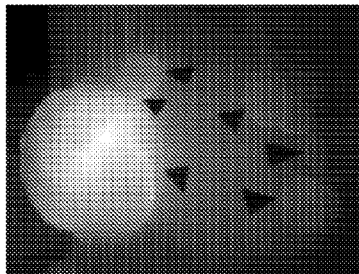
pxint1, Cy-5ex, Cy5em
