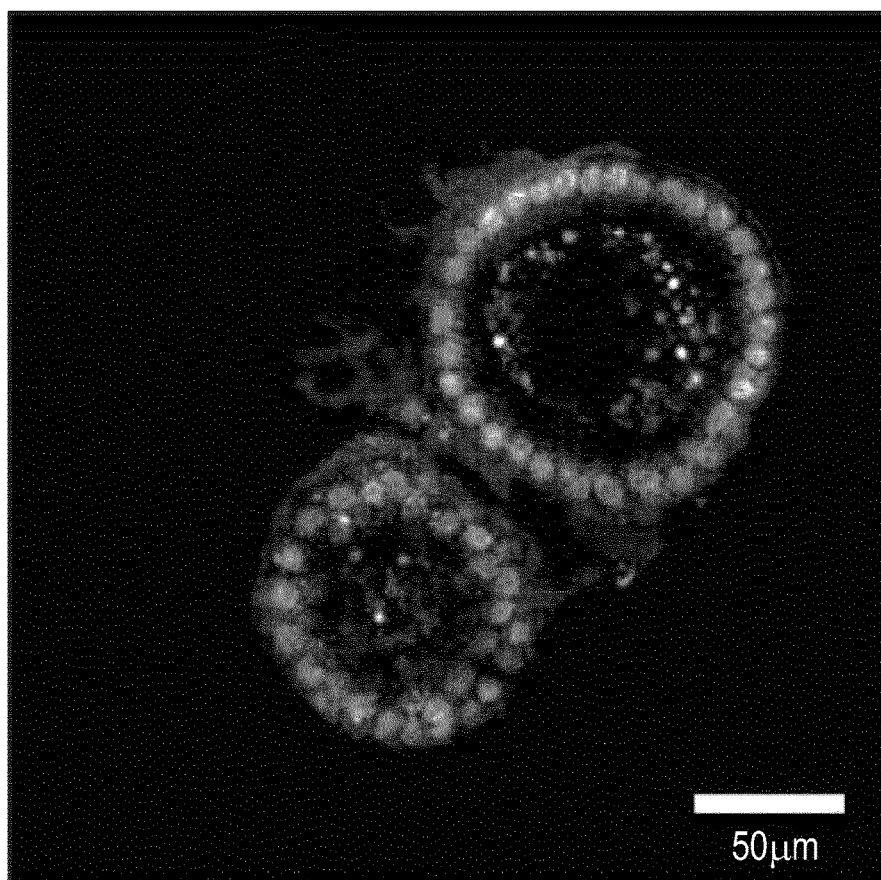
FIG. 16E + IDMI -EGF
