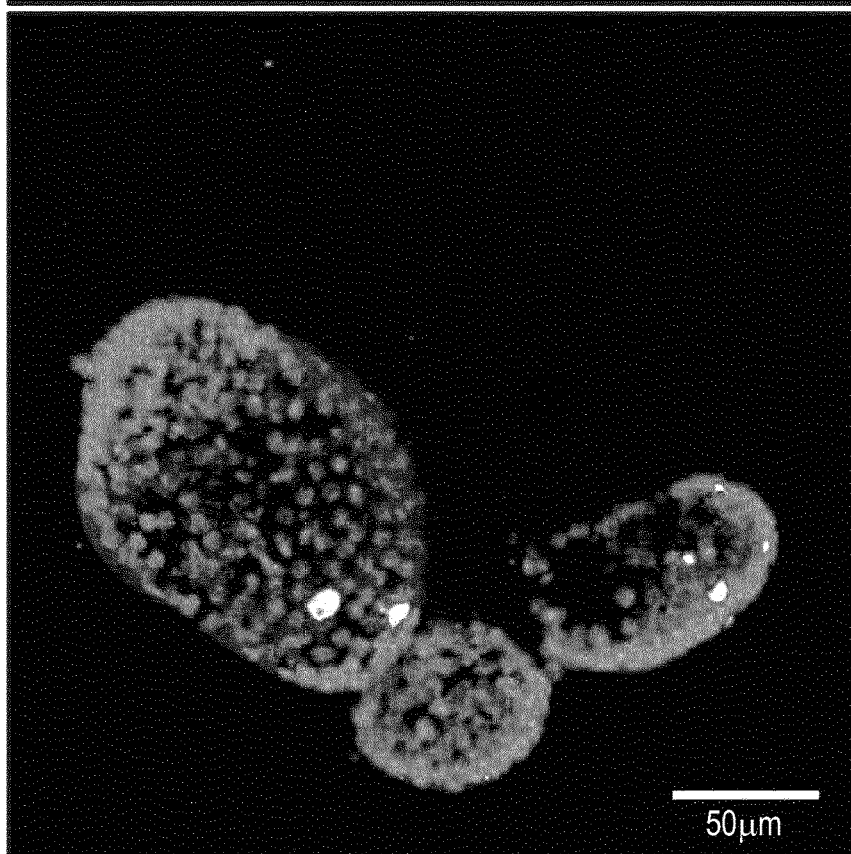
FIG. 13F IDMI TGFBi
