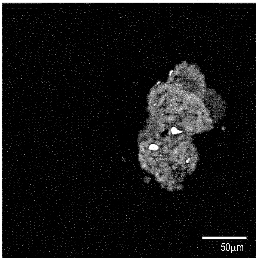
FIG. 13E IDMI MHY1485
