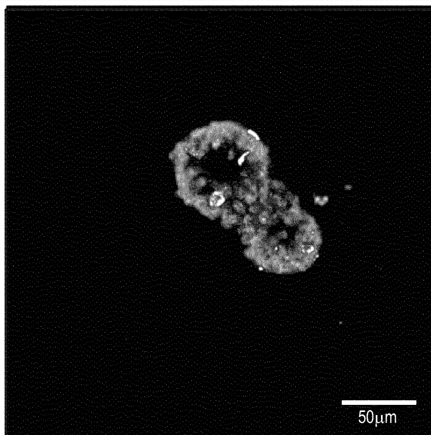
FIG. 13D IDMI Vismogenib
