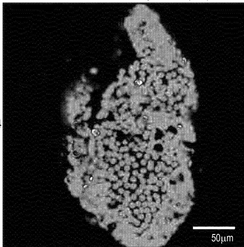
FIG. 13C IDMI -noggin BMP4
