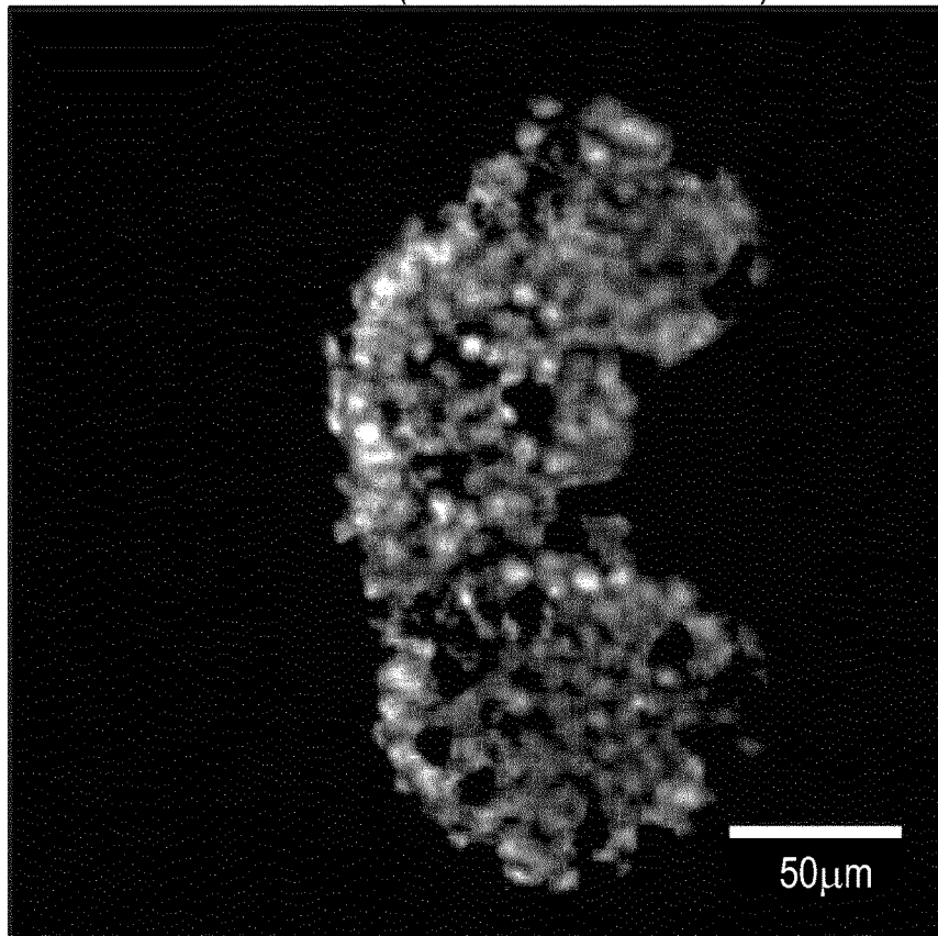
FIG. 14C IDMI -noggin BMP4
