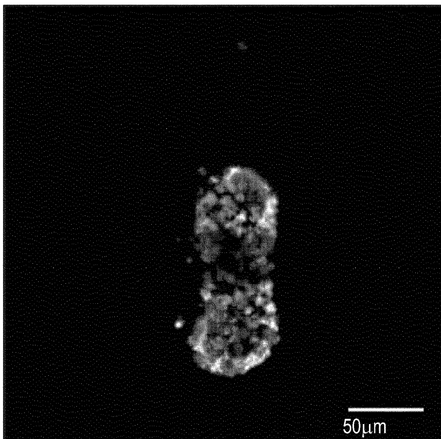
FIG. 14F IDMI TGFBi
