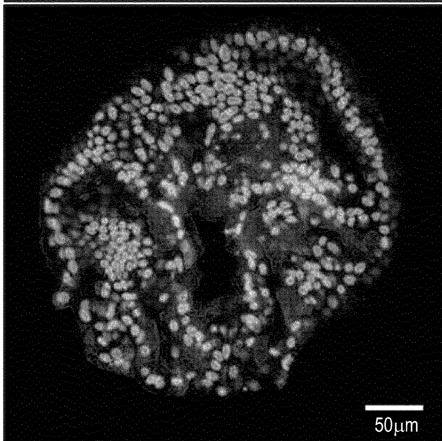
FIG. 16F + IDBMP4 -EGF/noggin
