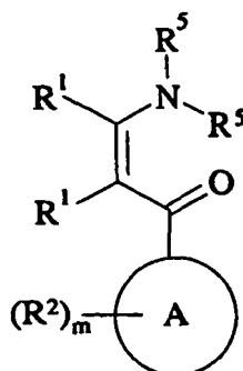
(VII)
