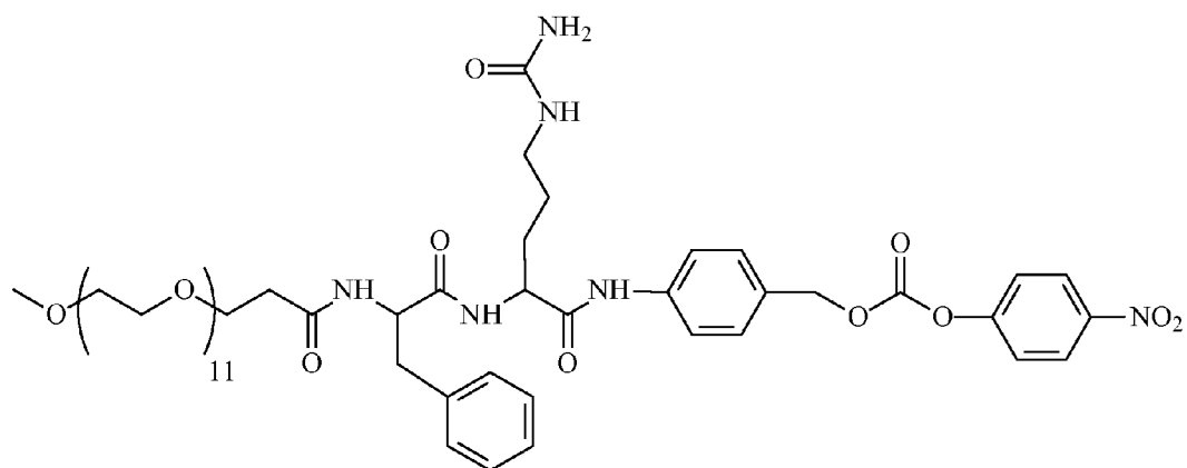
PEG 12 -Phe-Cit-PABC-PNP
