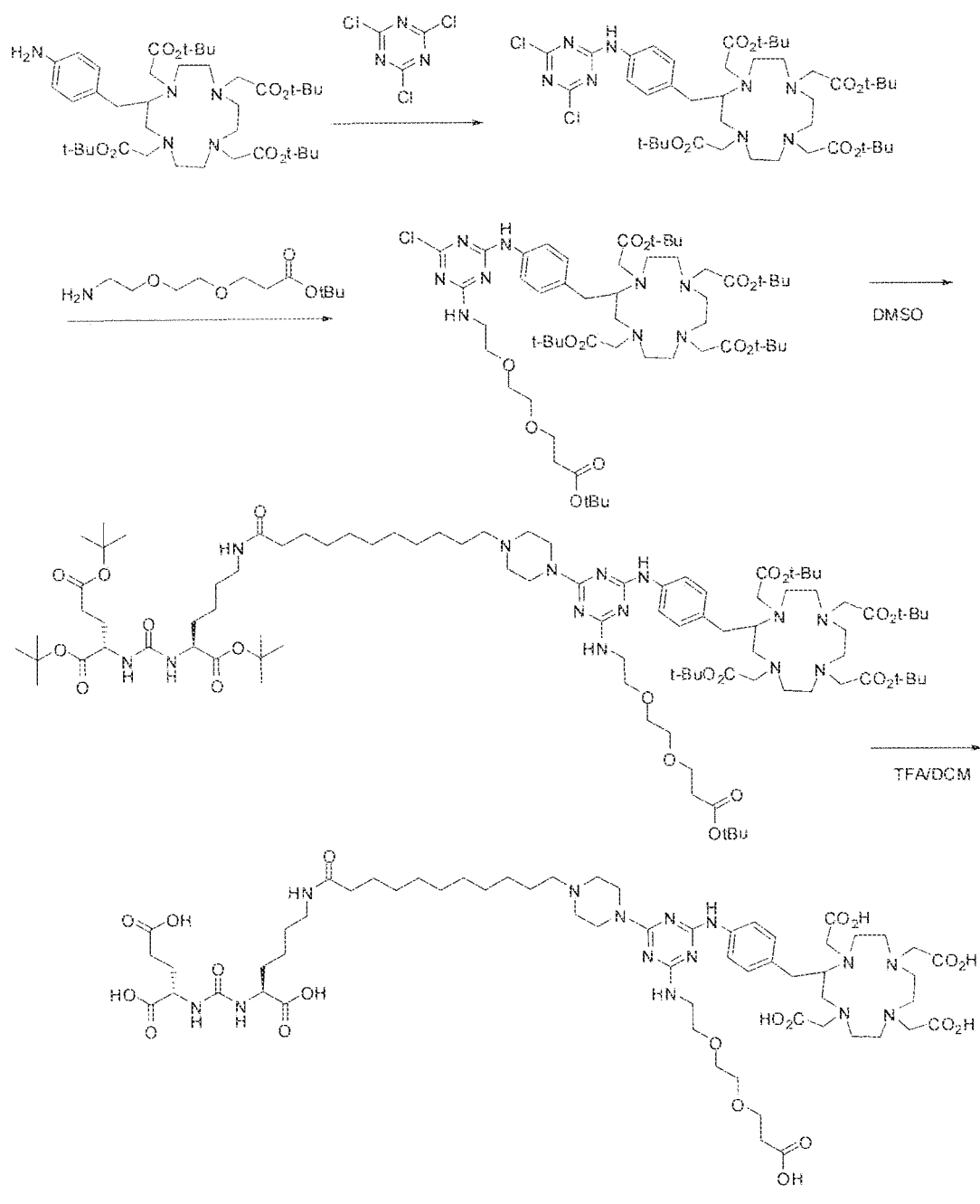
Scheme A.
