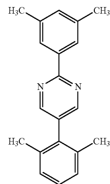
Hdmppm2-dmp
