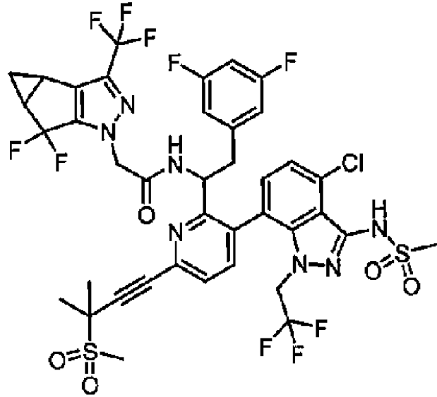
(Ia)
