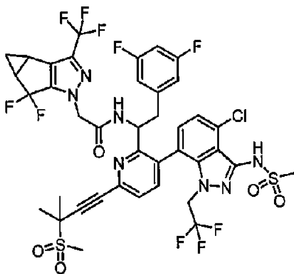
(Ia)
