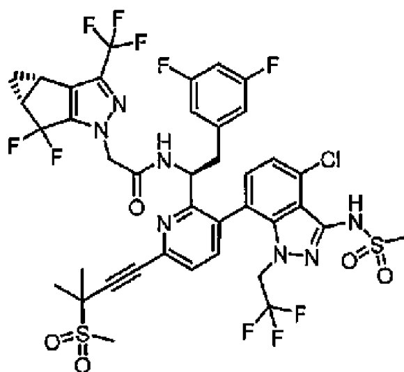
(Ib)
