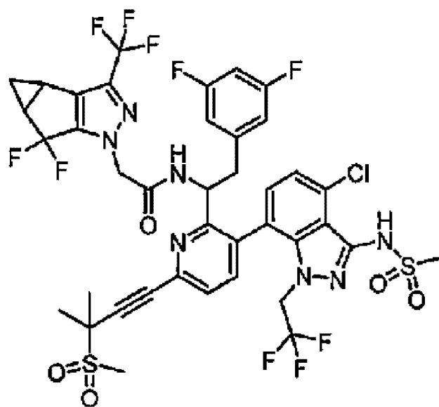
(Ia)
