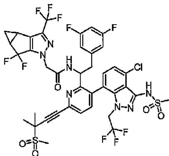
(Ia)
