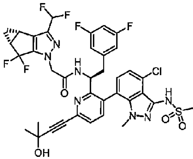
化合物A
