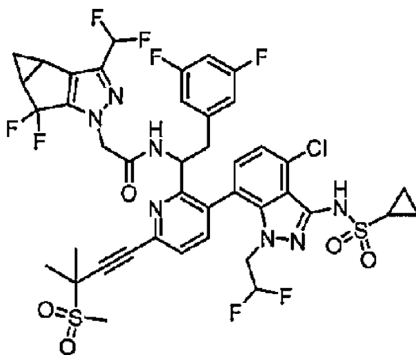
(IIa)
