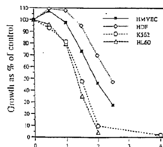
A4 Prodrug (nM) FIG. 2B
