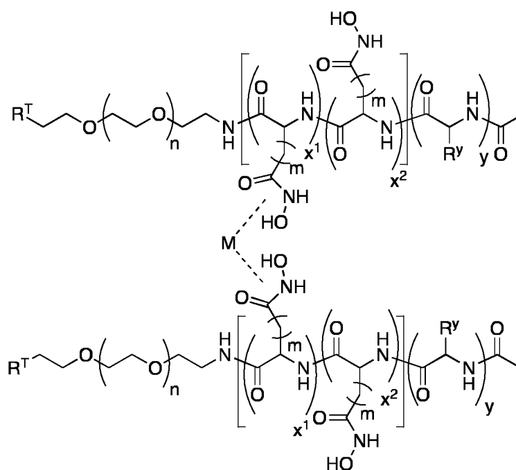
VII,
