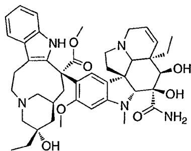
Vindesine
