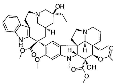
Vinblastine
