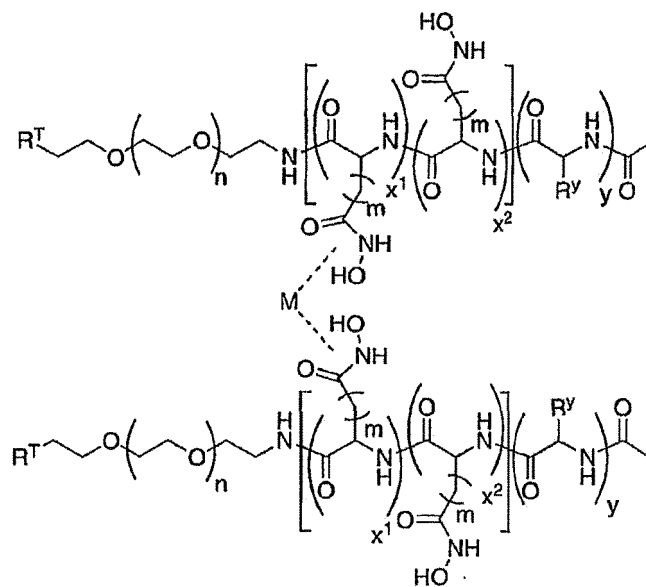
VII
