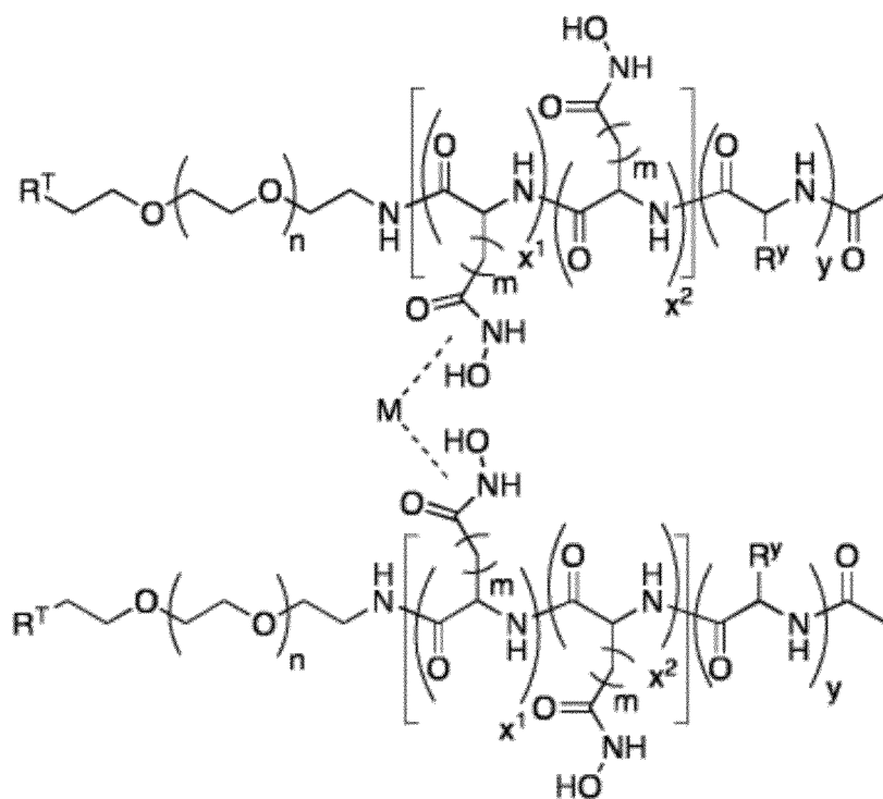
VII,
