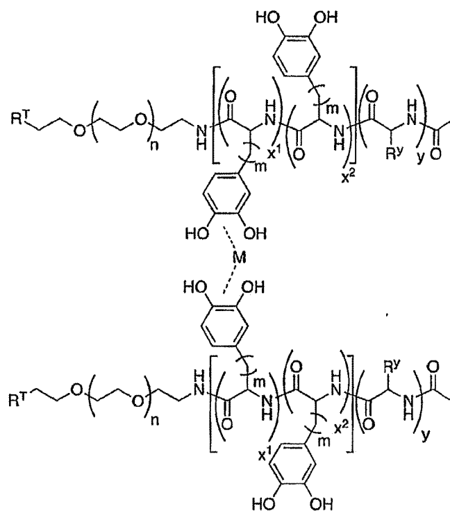
VIII
