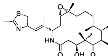
Ixepilone
