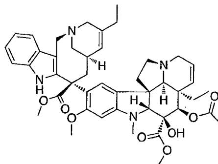
Vinorelbine
