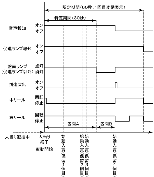
時短中タイミングチャート(特1保留なし)
