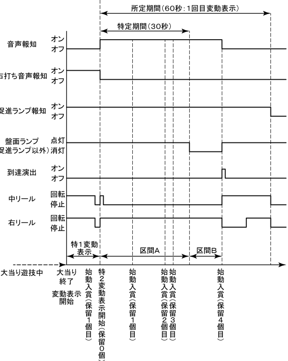
時短中タイミングチャート(特1保留あり)
