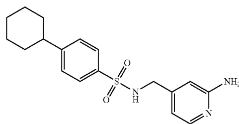
N-((2-aminopyridin-4-yl)methyl)-4-cyclohexylbenzenesulfonamide
