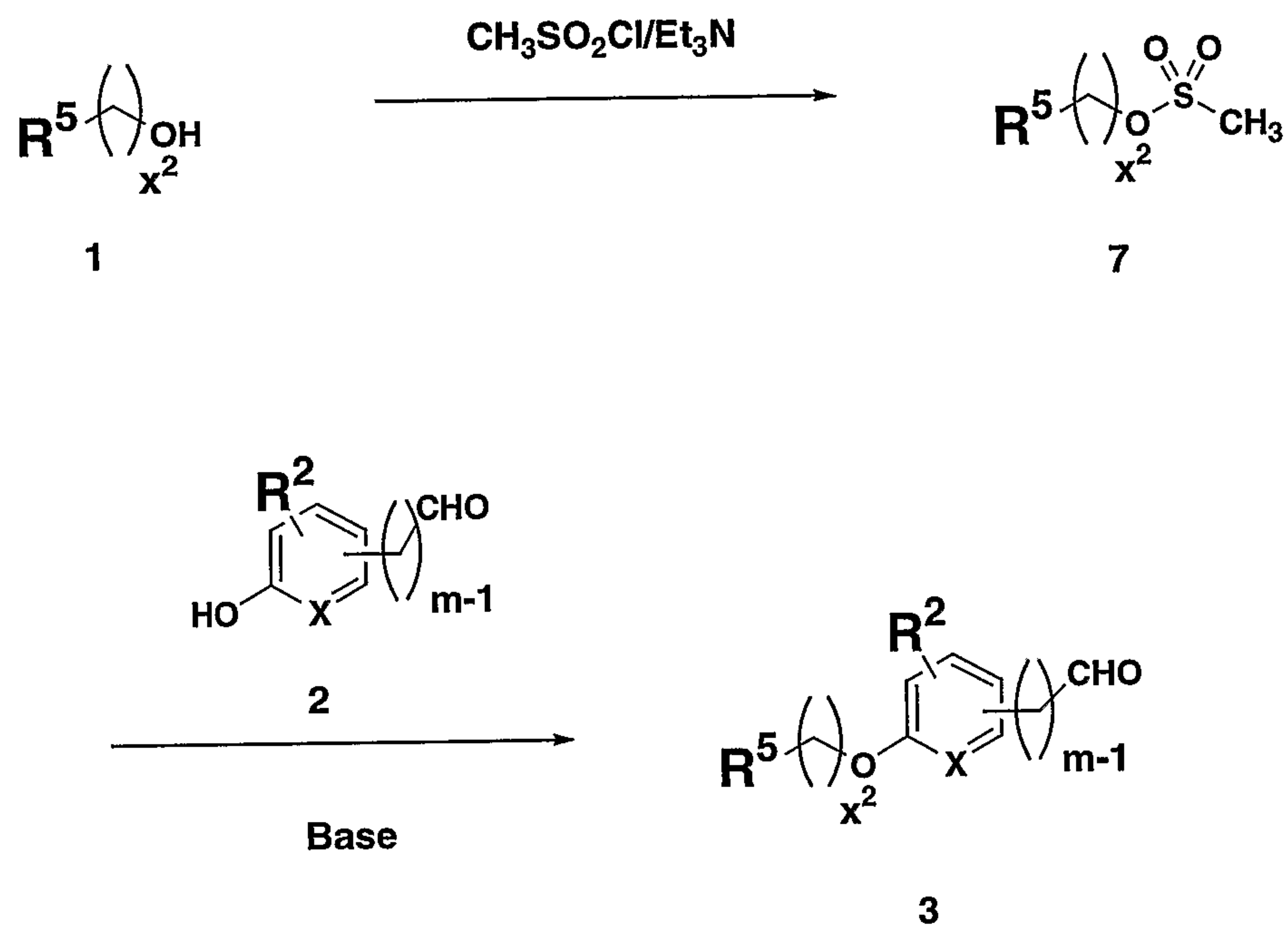
SCHEME 1A
