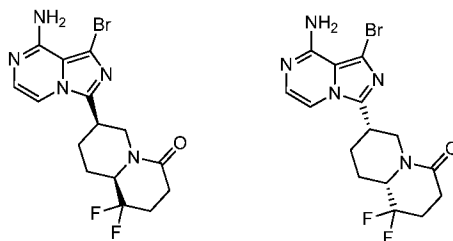
(7R,9aR)-7-(8-amino-1-bromoimidazo[1,5-a]pyrazin-3-yl)-1,1-difluorohexahydro-1H-quinolizin-4(6H)-one
