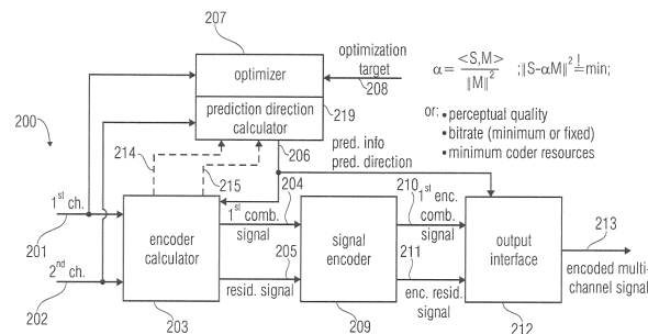
FIG 2 (AUDIO ENCODER)
