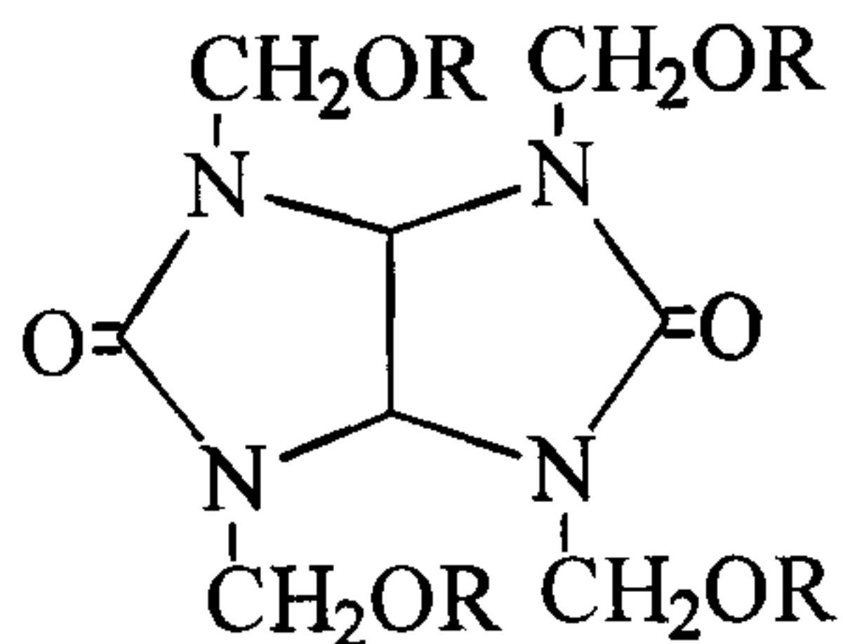
glycoluril
