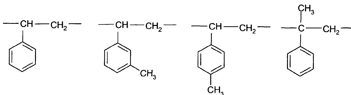
Struktureinheit III
