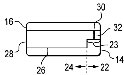
SECTION A-A FIG. 1C
