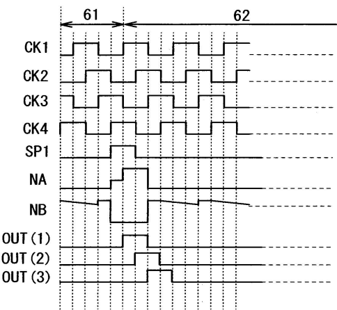
도면13
