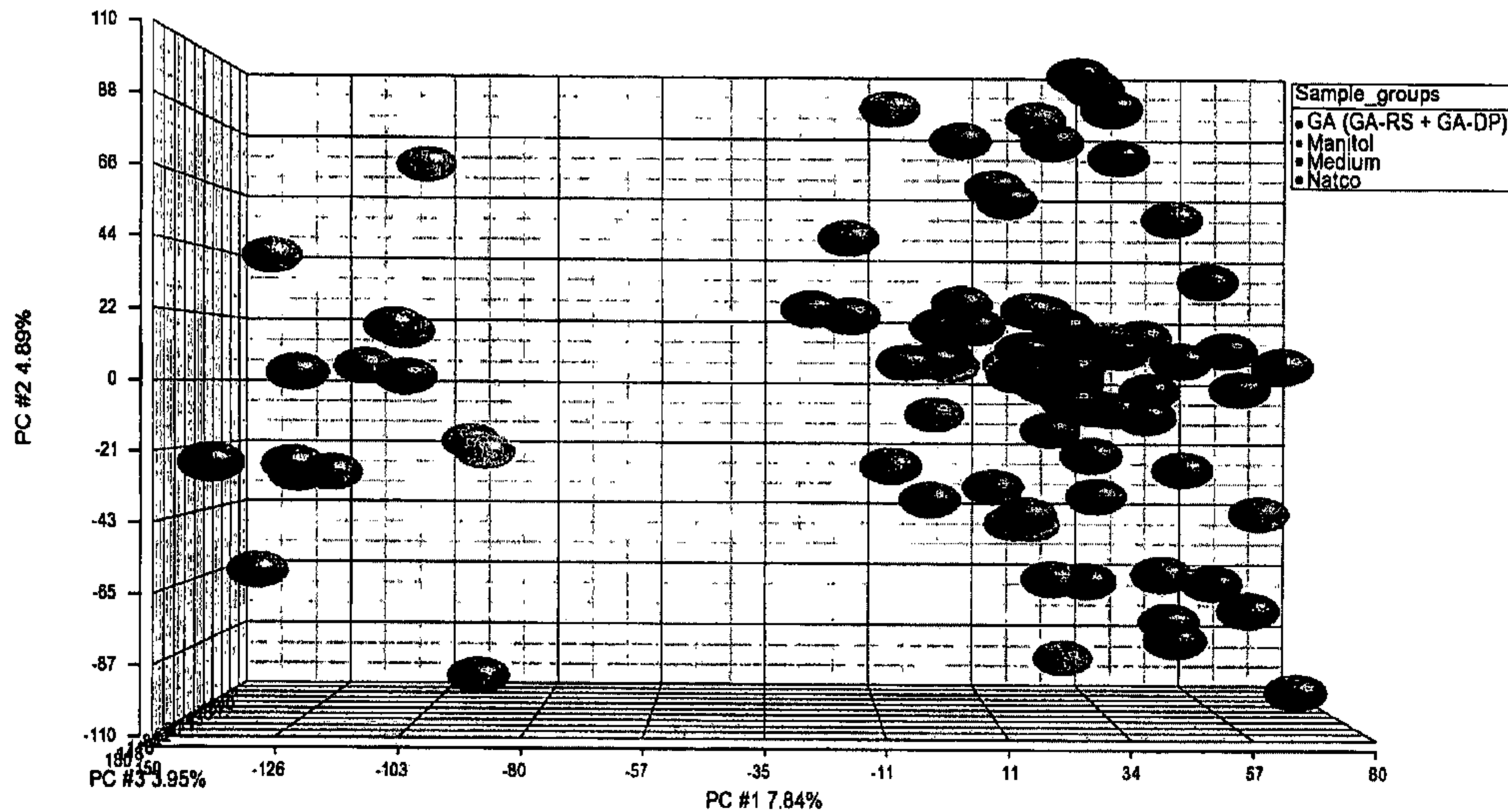
PCA Mapping (16.7%)
