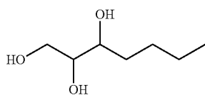
1,2,3-Heptanetriol
