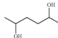
2,5-Hexanediol
