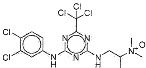
1-((4-((3,4-dichlorophenyl)amino)-6-(trichloromethyl)-1,3,5-triazin-2-yl)amino)-N,N-dimethylpropan-2-amine oxide
