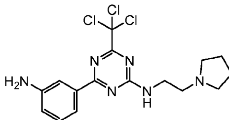
4-(3-aminophenyl)-N-(2-(pyrrolidin-1-yl)ethyl)-6-(trichloromethyl)-1,3,5-triazin-2-amine
