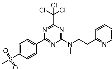
N-methyl-4-(4-(methanesulfonyl)phenyl)-N-(2-(pyridin-2-yl)ethyl)-6-(trichloromethyl)-1,3,5-triazin-2-amine
