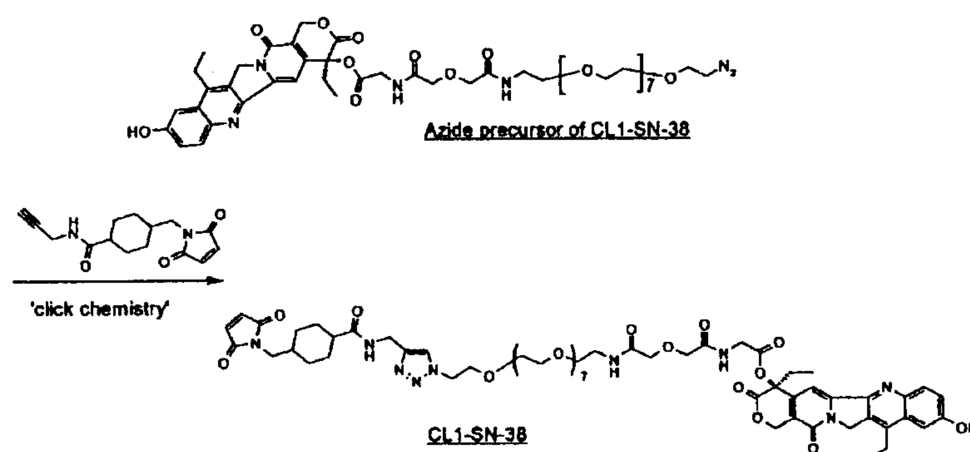
Scheme-1
