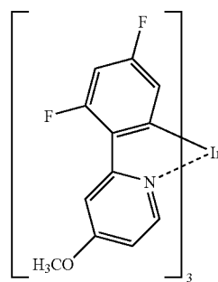
(K-1)
