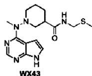
1-[Метил-[7Н-пиррол[2,3-d]пиримидин-4-]амино]-N-(метилтиометил)пиперидил-3-формамид
