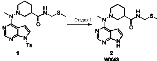
1-[Метил-[7Н-пиррол[2,3-d]пиримидин-4-]амино]-N-(метилтиометил)пиперидил-3-формамид
