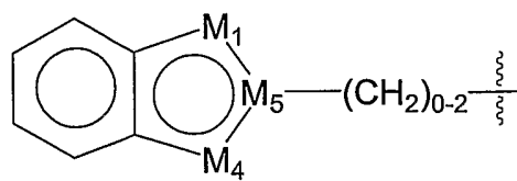
(IIIb)
