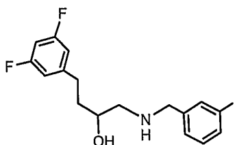
EXAMPLE 199: 1-(4-AMINO-BENZYLAMINO)-4-(3,5-DIFLUORO-PHENYL)-BUTAN-2-OL
