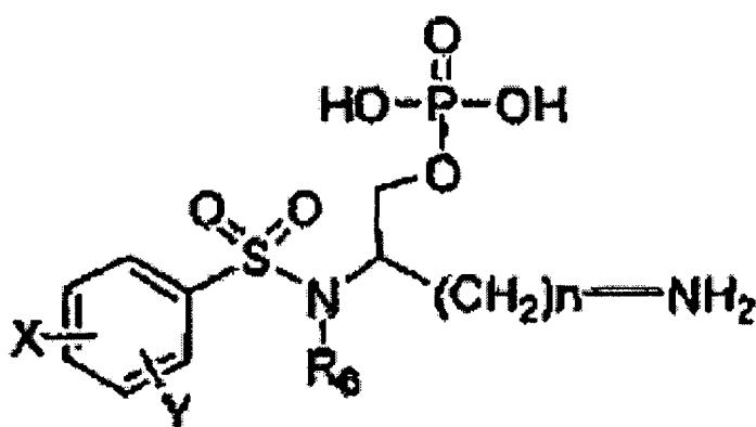
XIV
