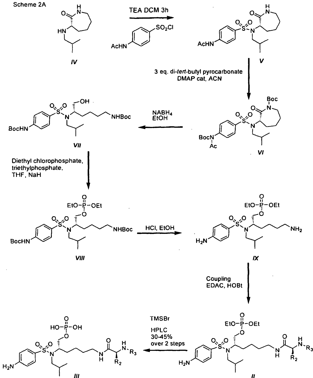
Scheme 2A
