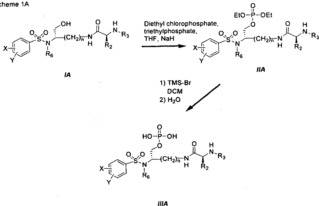
Scheme 1A
