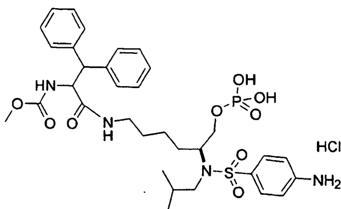
IIIB
