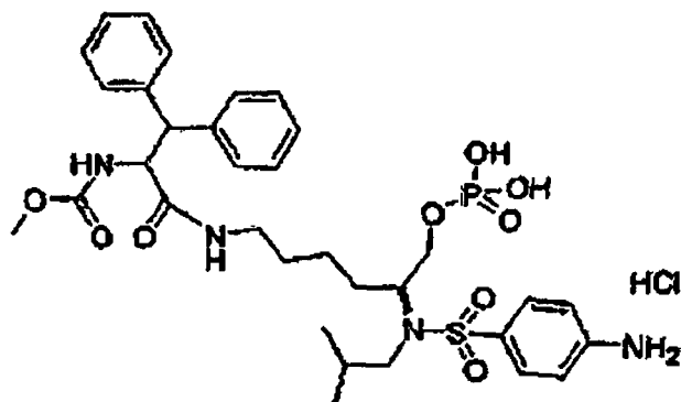
III B
